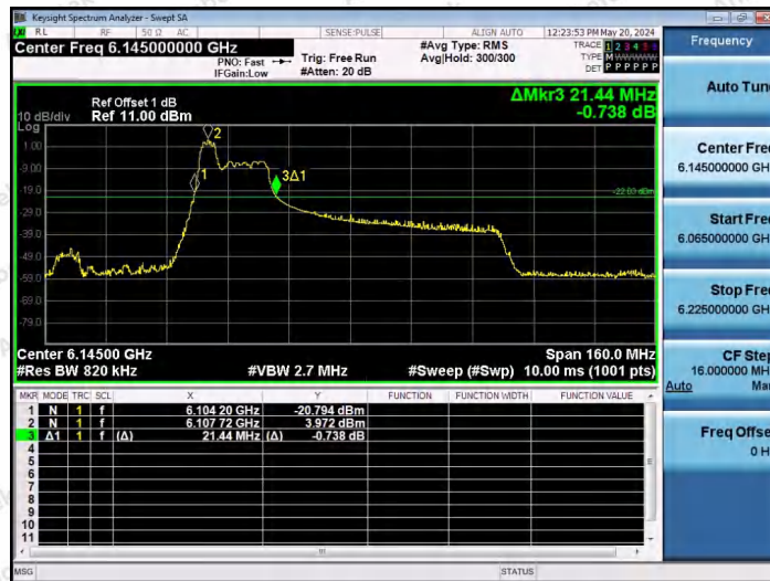
11AX80SISO-Ant1-6145-52Tone-RU37
