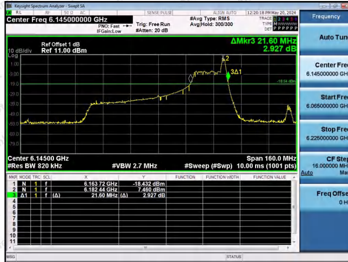
11AX80SISO-Ant1-6145-26Tone-RU36
