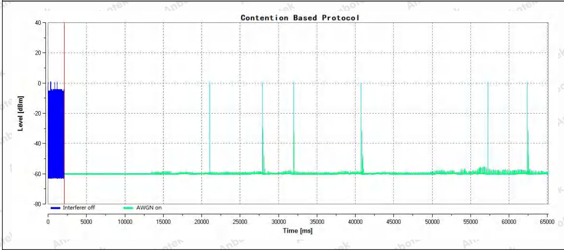
11AX80SISO-Ant1-6465-6465-PASS
