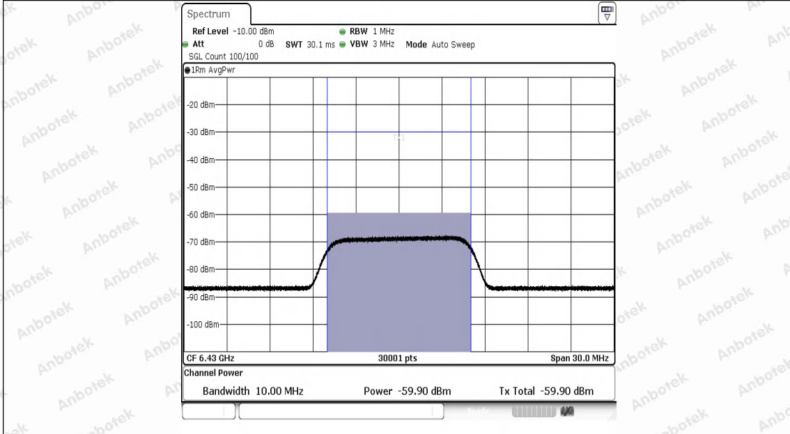
11AX80SISO-Ant1-6465-6430-PASS
