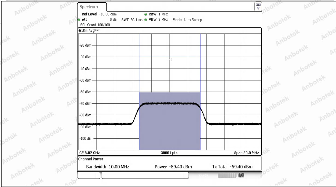
11AX80SISO-Ant1-5985-6020-PASS
