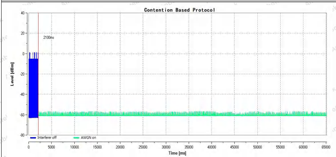
11AX80SISO-Ant1-6865-6865-PASS
