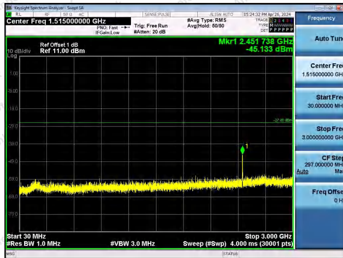
11AX80SISO-Ant1-6145-30~3000-PASS
