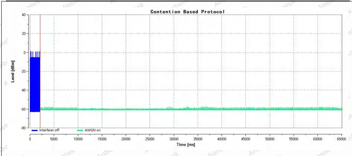
11AX80SISO-Ant1-5985-6020-PASS
