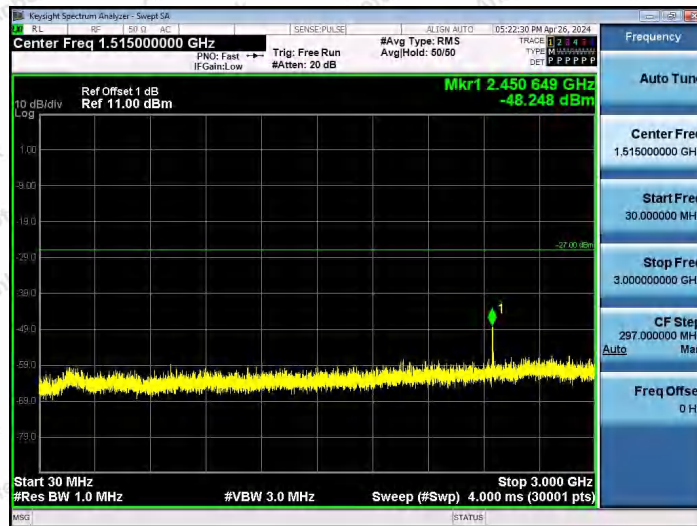
11AX80SISO-Ant1-5985-30~3000-PASS
