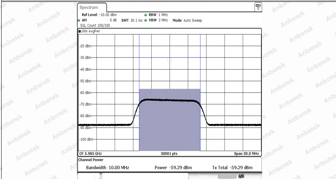
11AX80SISO-Ant1-5985-5950-PASS
