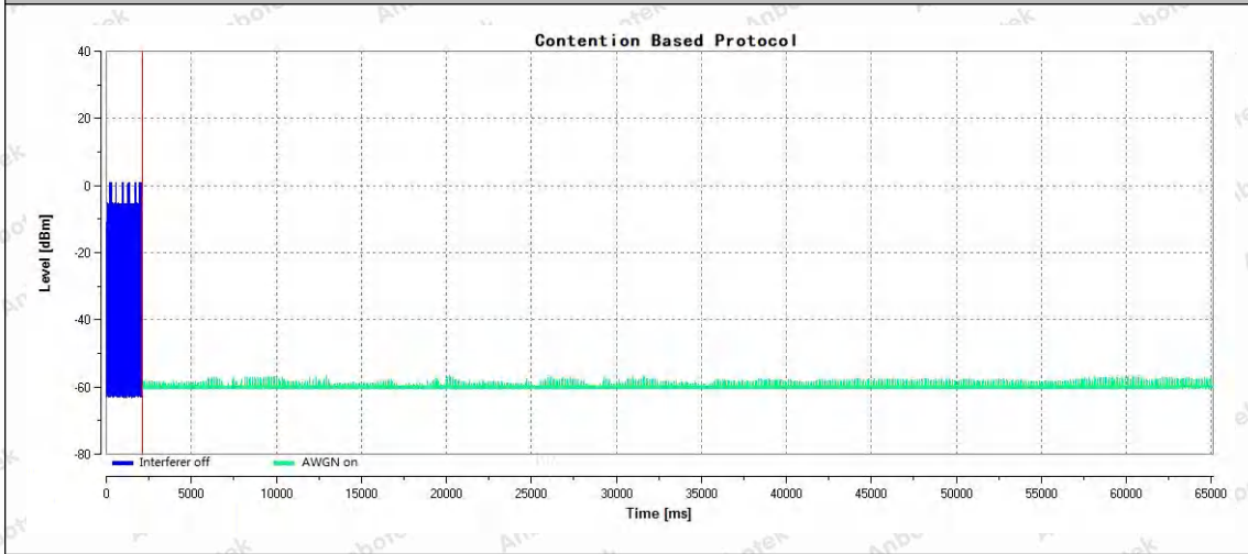
11AX80SISO-Ant1-5985-5950-PASS
