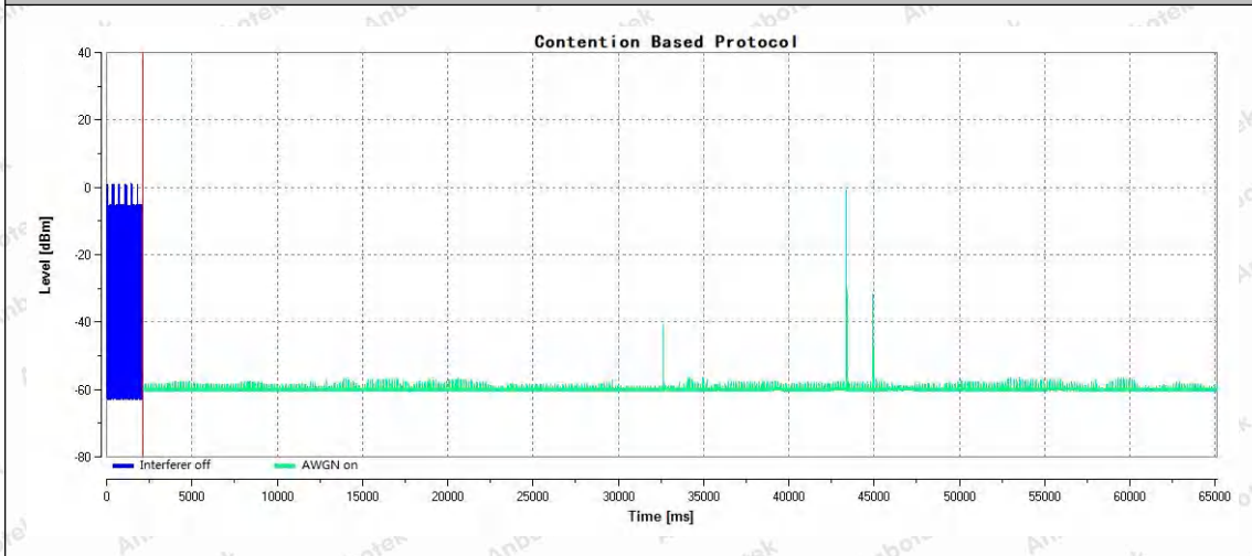
11AX80SISO-Ant1-5985-5985-PASS
