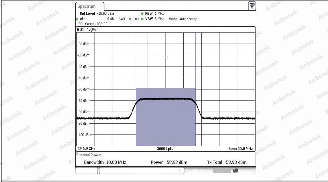
11AX80SISO-Ant1-6865-6900-PASS
