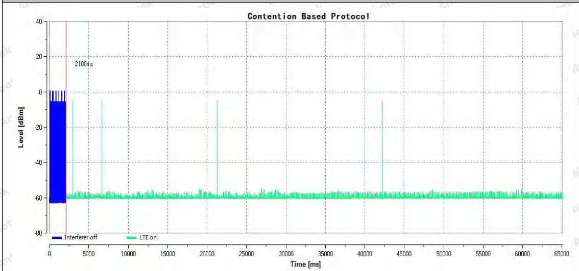
11AX80SISO-Ant1-6865-6830-PASS
