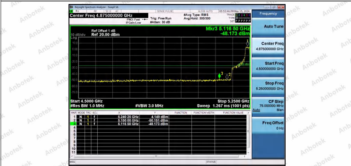
11AX80SISO-Ant1-5210-242Tone-RU64-PASS
