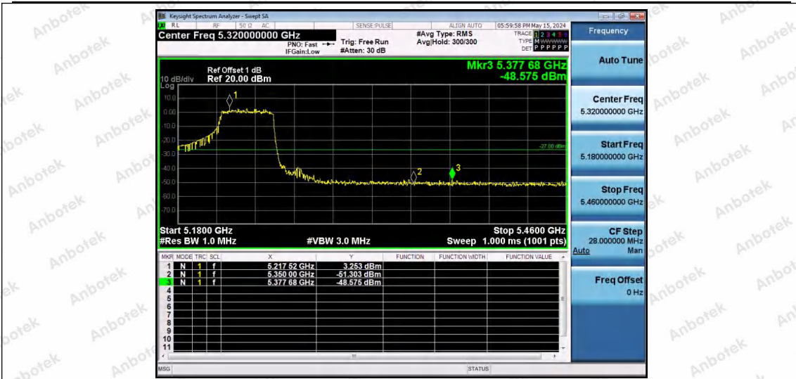
11AX80SISO-Ant1-5210-484Tone-RU66-PASS
