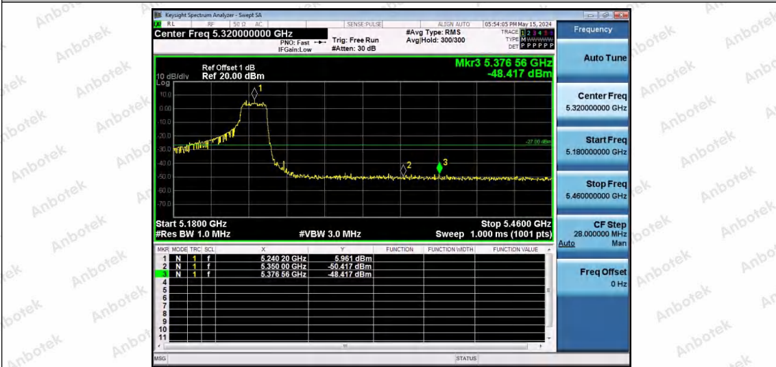
11AX80SISO-Ant1-5210-242Tone-RU64-PASS
