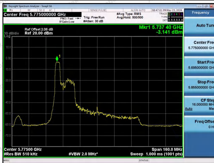
11AX80SISO-Ant1-5775-52Tone-RU37-PASS
