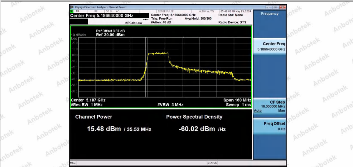
11AX80SISO-Ant1-5210-242Tone-RU61-PASS
