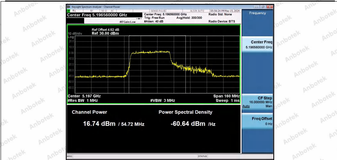
11AX80SISO-Ant1-5210-484Tone-RU65-PASS
