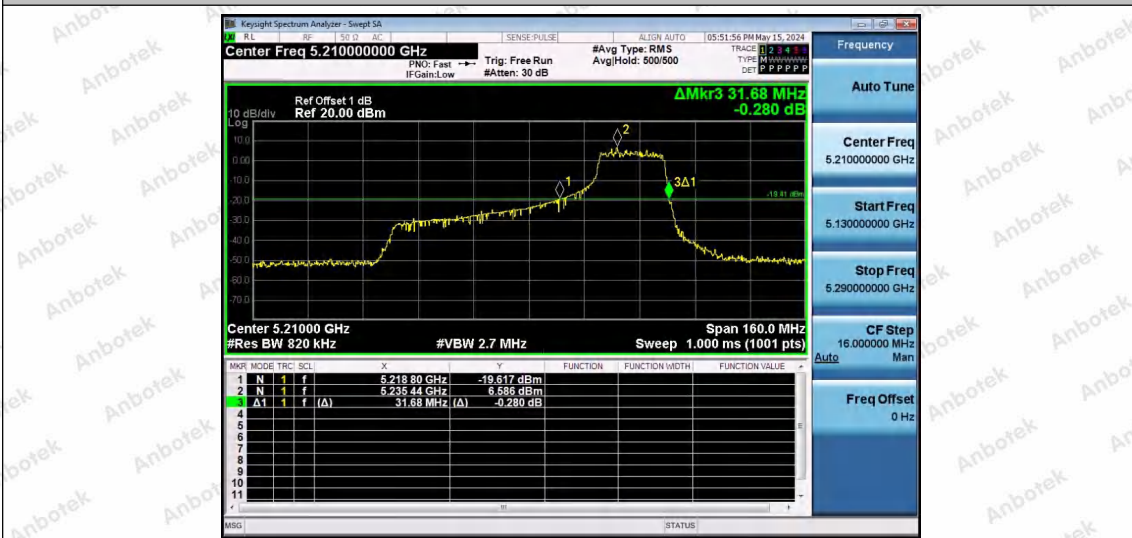
11AX80SISO-Ant1-5210-242Tone-RU64
