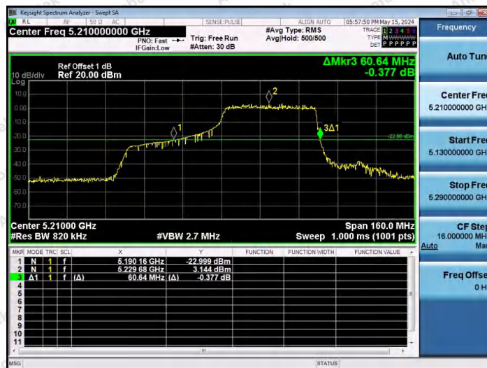
11AX80SISO-Ant1-5210-484Tone-RU66
