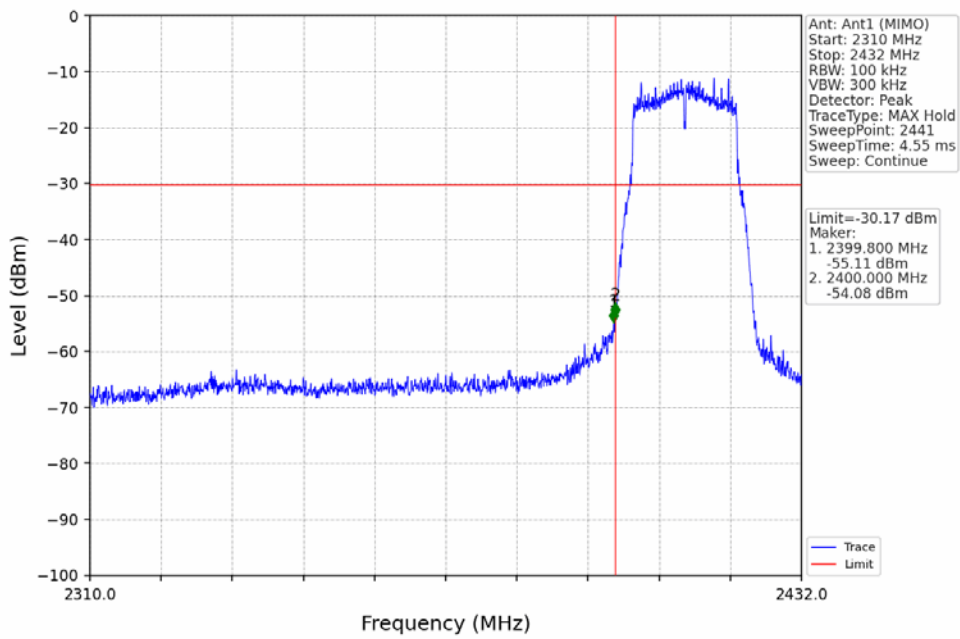
802.11n(HT20)_LCH_2412MHz_Ant1 (MIMO)_NTNV
