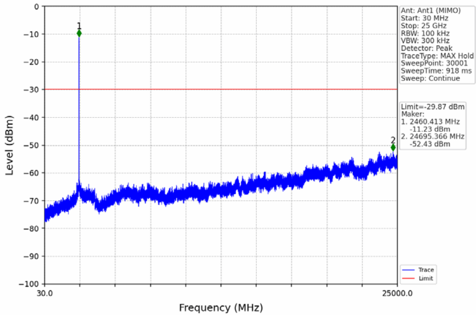
802.11n(HT20)_HCH_2462MHz_Ant1 (MIMO)_NTNV
