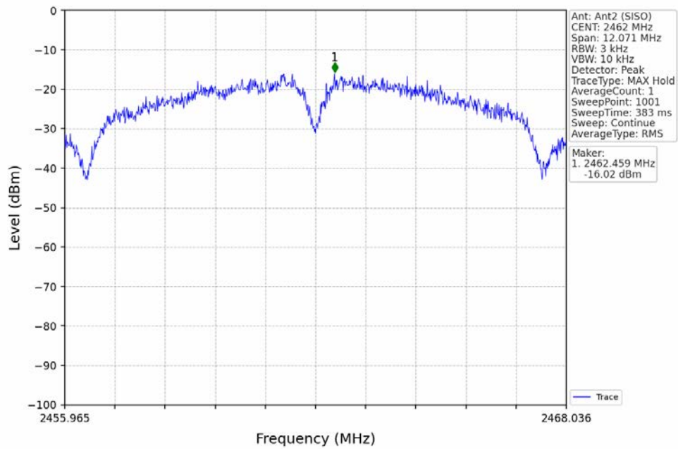
802.11b_HCH_2462MHz_Ant2 (SISO)_NTNV
