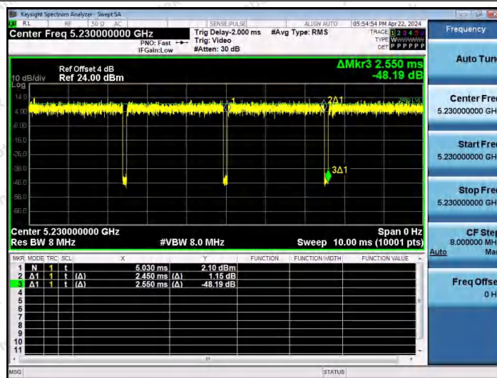
NTNV-11AX40MIMO-Ant1-5230
