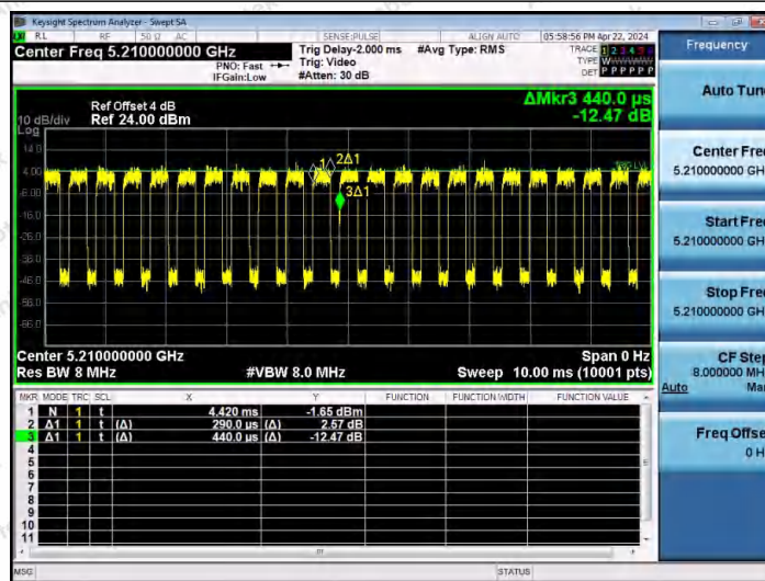
NTNV-11AX80MIMO-Ant1-5210
