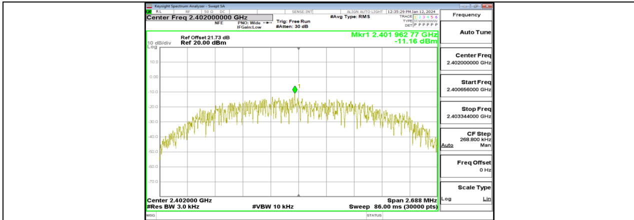
LE 2M_Ant1_2402
