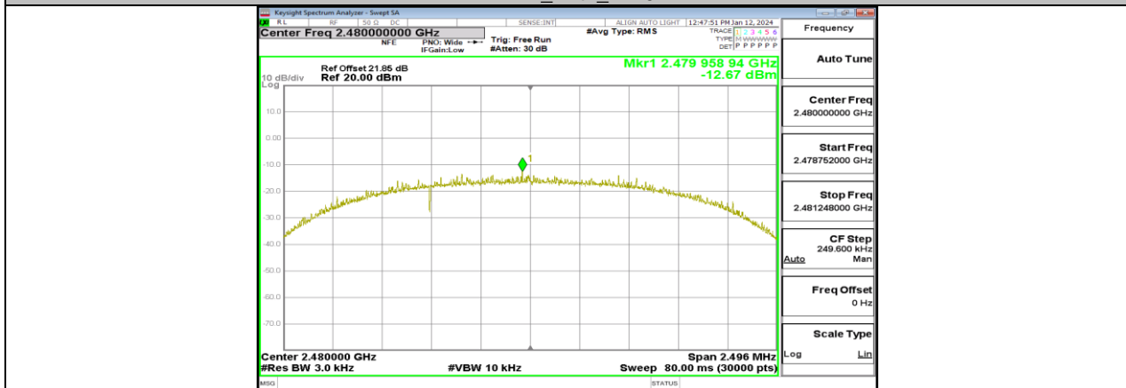
LE 2M_Ant1_2480
