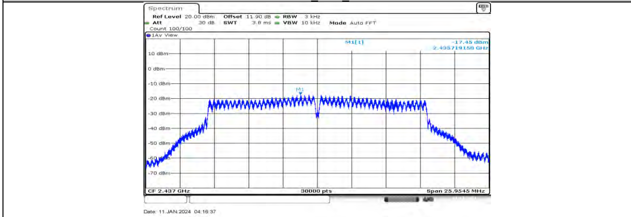
11G-CDD Ant2 2437
