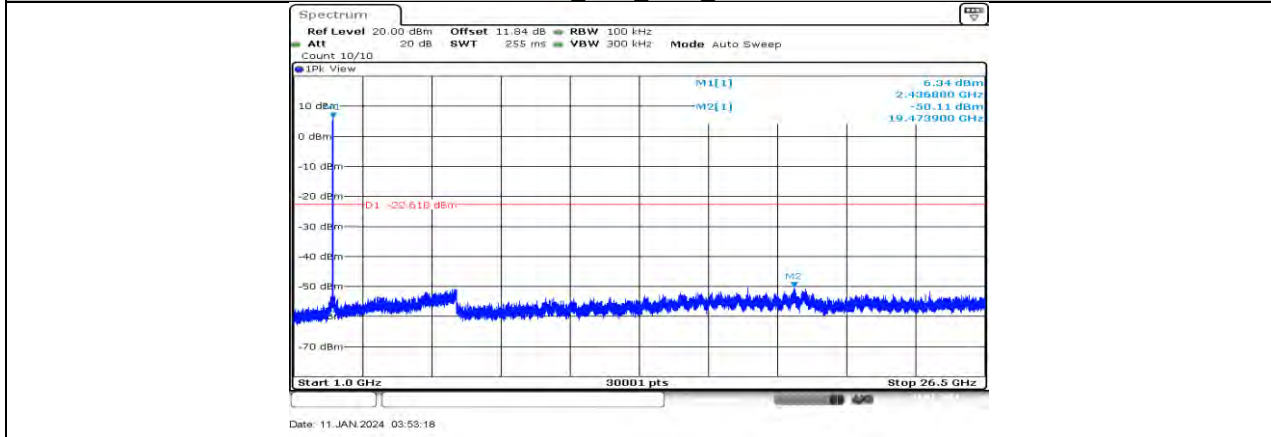
11B-CDD Ant2 2437 1000~26500
