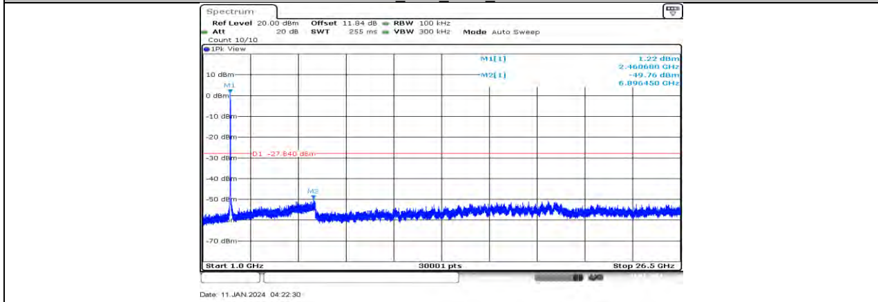
11G-CDD Ant1 2462 1000~26500
