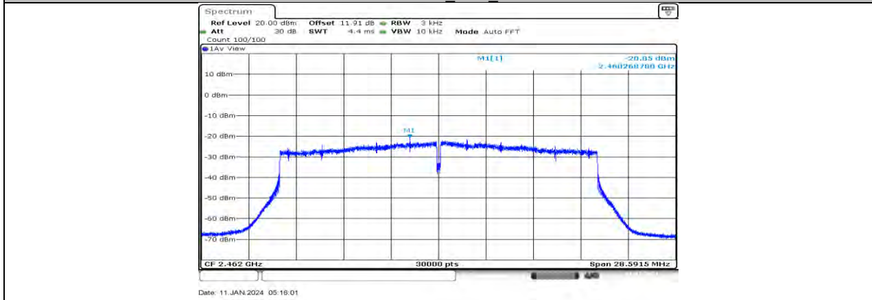
11AX20MIMO_Ant2_2462
