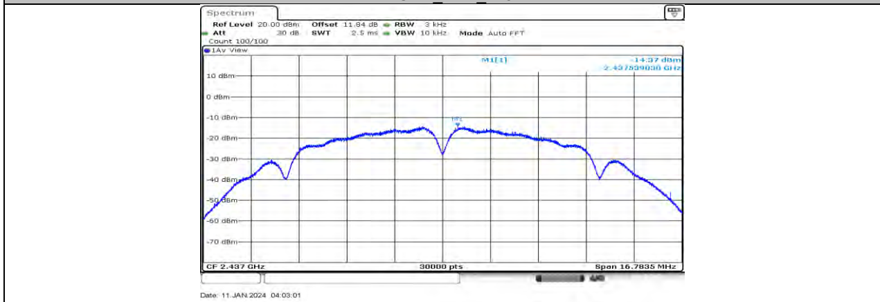
11B-CDD Ant2 2437
