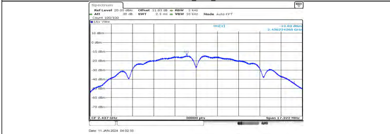
11B-CDD Ant1 2437
