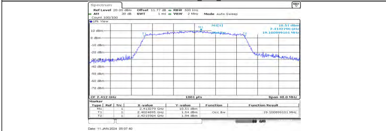
11AX20MIMO Ant2_2412
