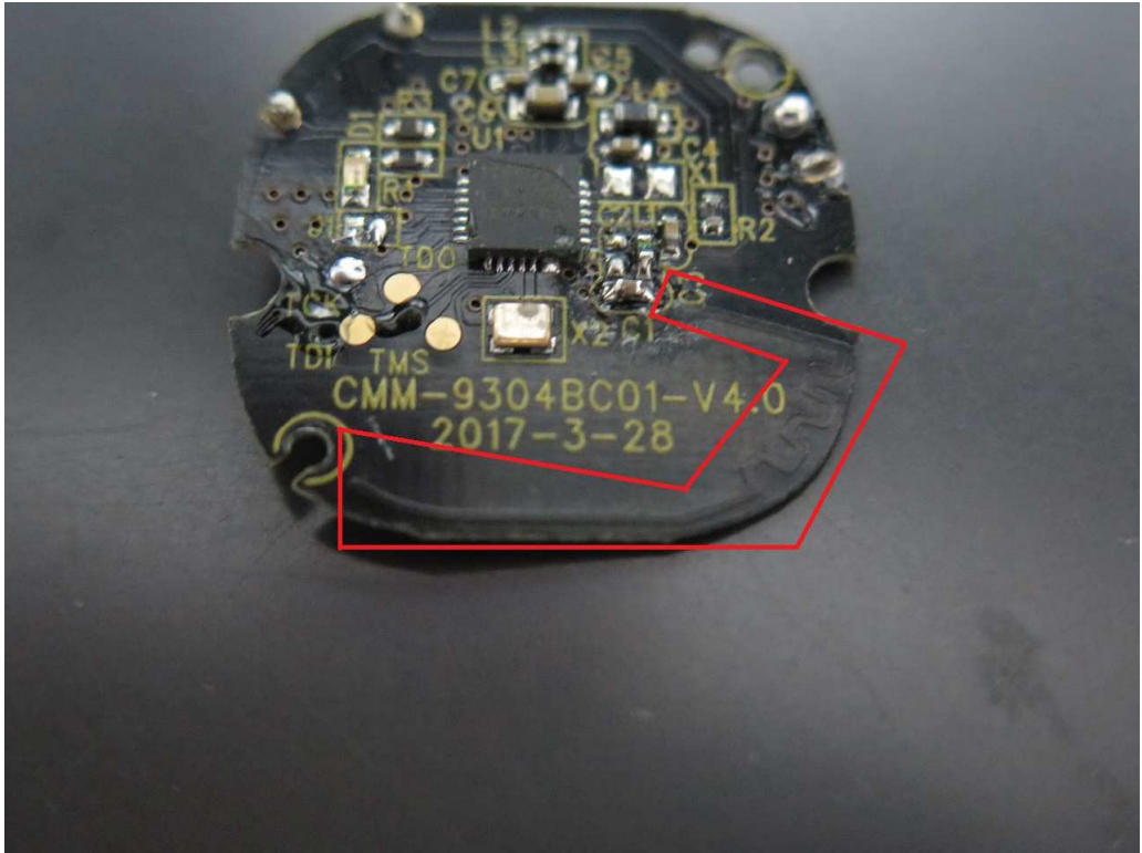
EUT Antenna
