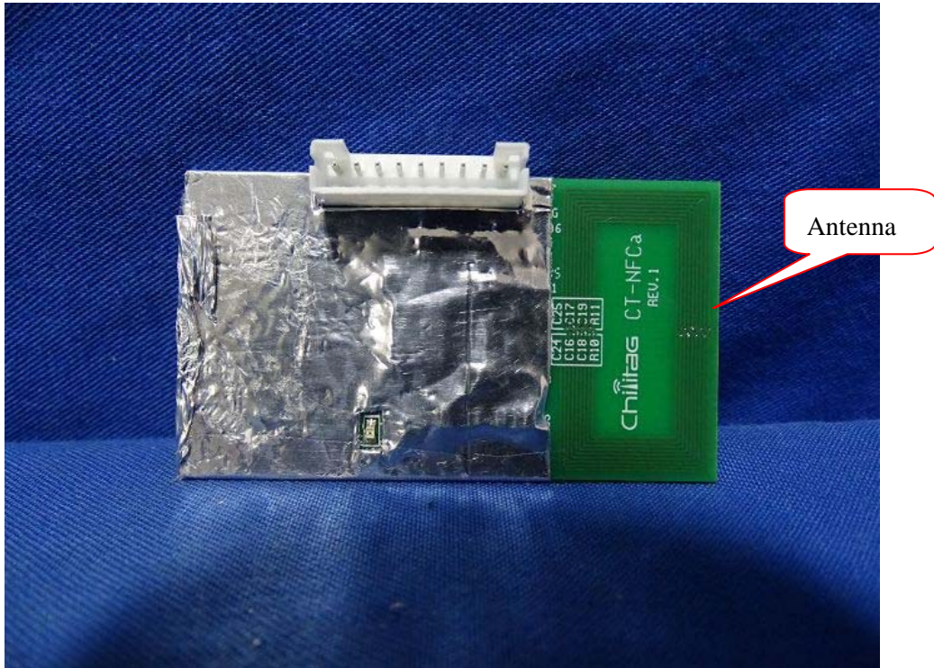
(15) EUT Photo
