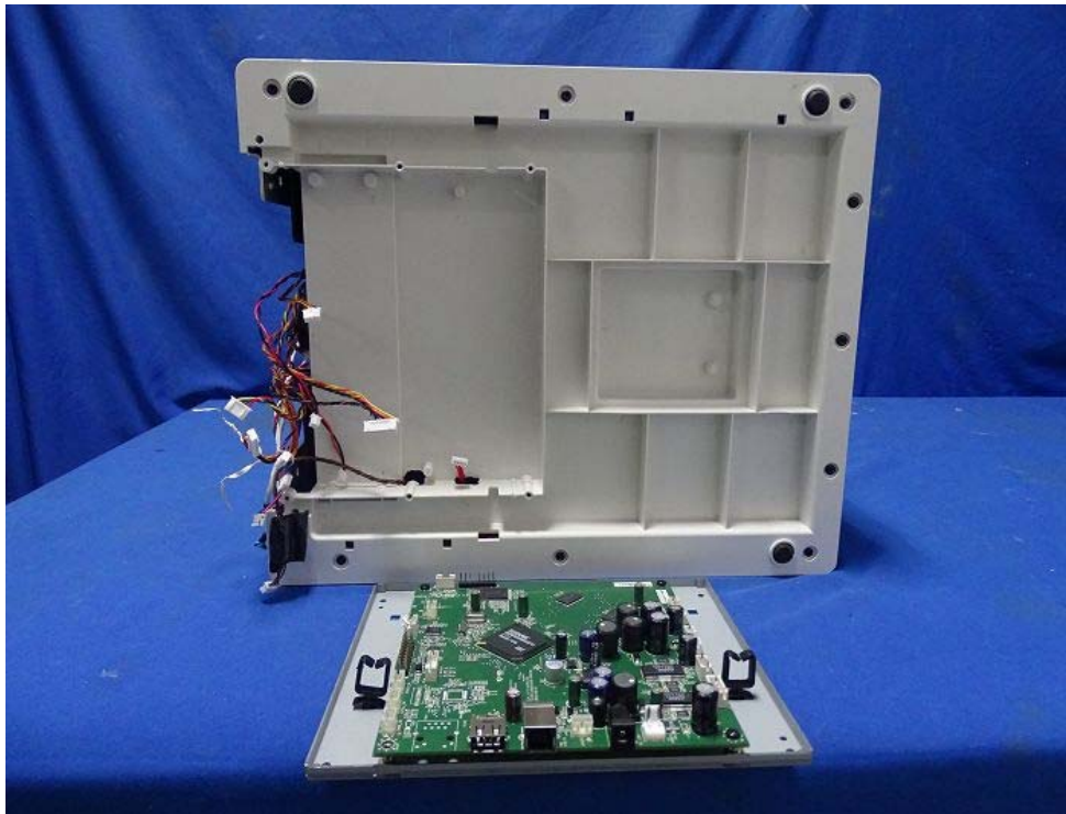
(6) EUT Photo
