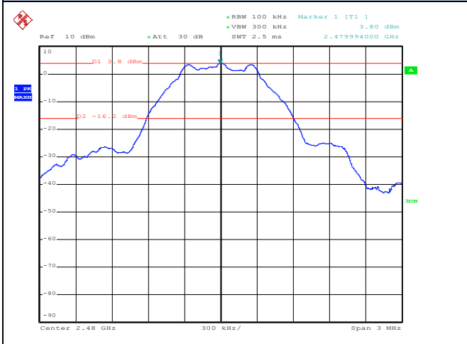
2479 – 2481 MHz
