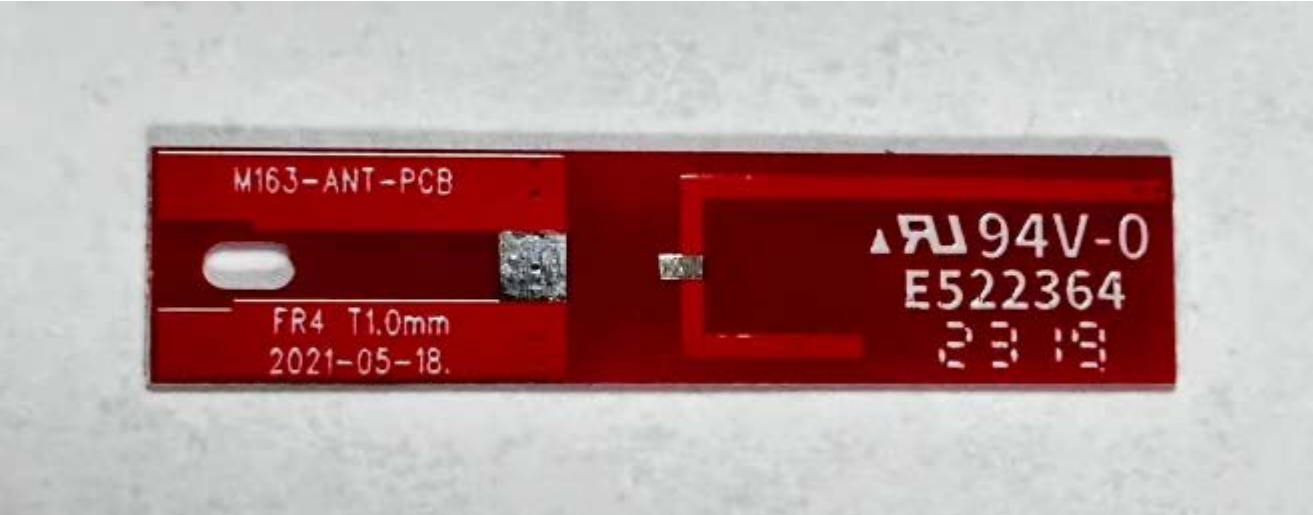
天线图片 Antenna Picture
