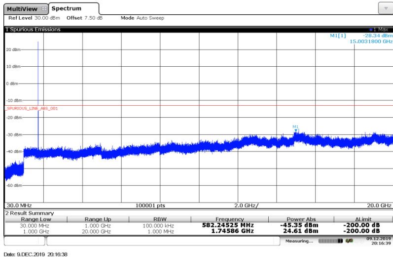
Band4-10MHz-QPSK-20350-1RB#
