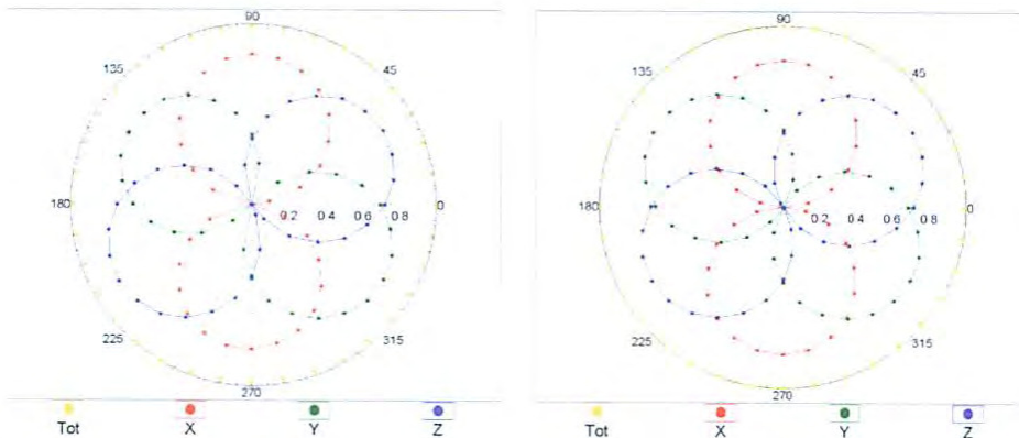
f=1800 MHz,R22
