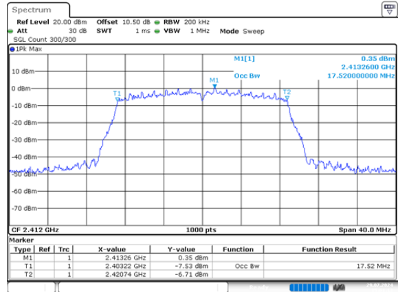
n20_2412MHz_Chain 1 17.520MHz
