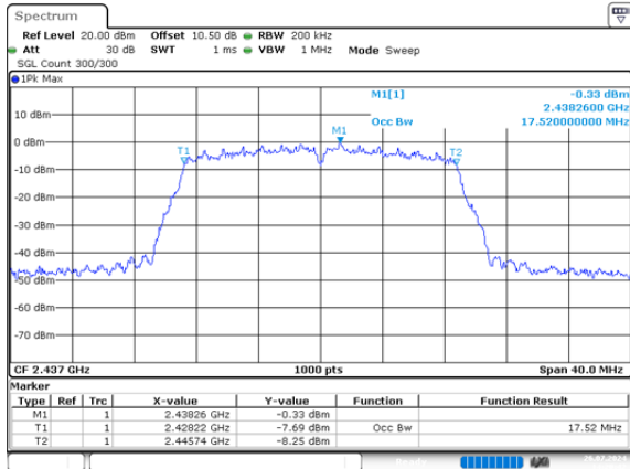
n20_2437MHz_Chain 0 17.520MHz
