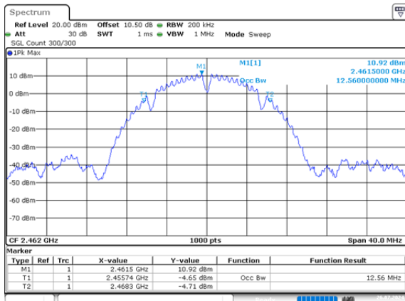
b_2462MHz_Chain 0 12.560MHz
