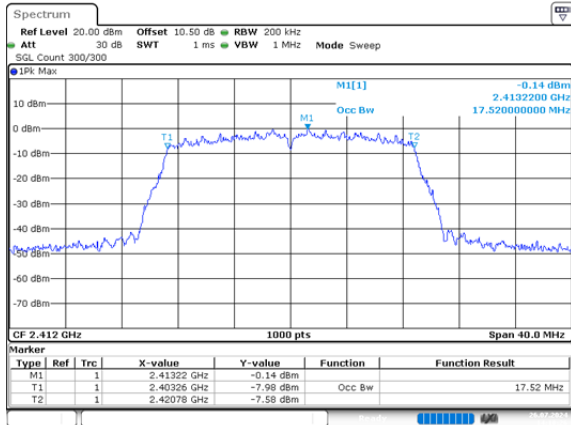
n20_2412MHz_Chain 0 17.520MHz
