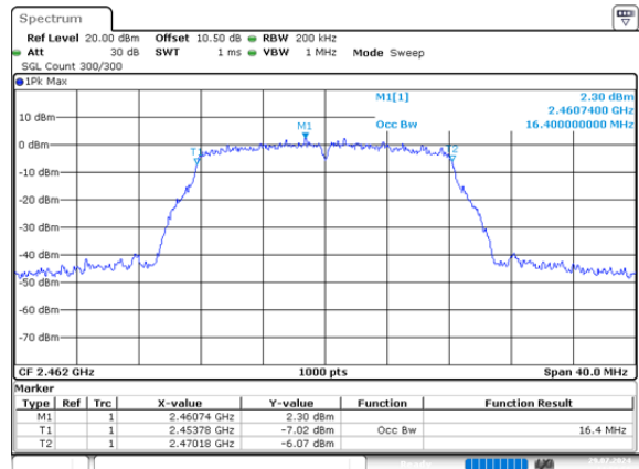
g_2462MHz_Chain 1 16.400MHz
