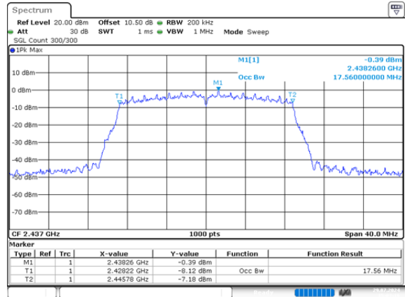
n20_2437MHz_Chain 1 17.560MHz
