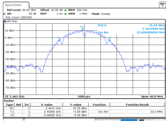
b_2462MHz_Chain 1 12.600MHz
