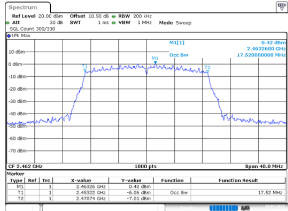
n20_2462MHz_Chain 1 17.520MHz
