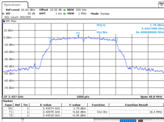
g_2437MHz_Chain 0 16.400MHz
