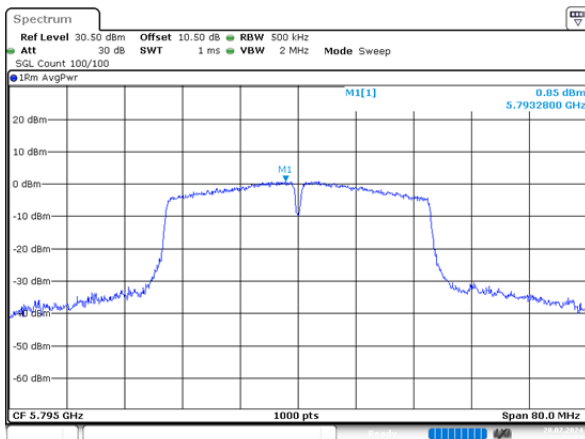
n40_5795MHz_Chain 0 0.85dBm/MHz
