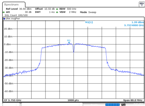
n40_5755MHz_Chain 1 1.39dBm/MHz
