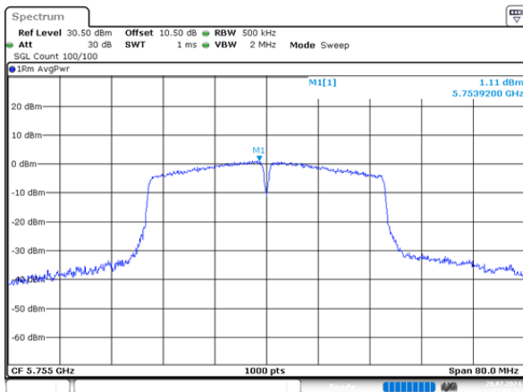
n40_5755MHz_Chain 0 1.11dBm/MHz
