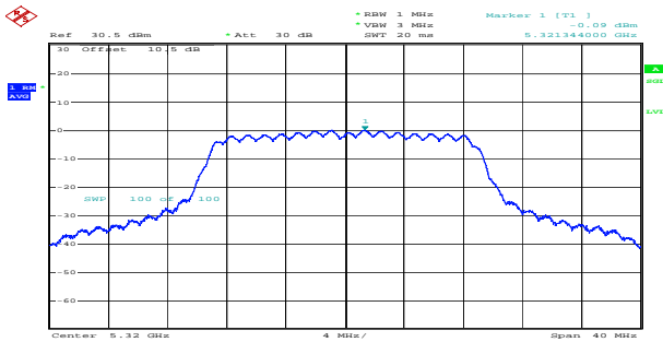
n20_5320MHz_Chain 0 -0.09dBm/MHz
