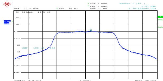
a_5700MHz_Chain 1 0.27dBm/MHz
