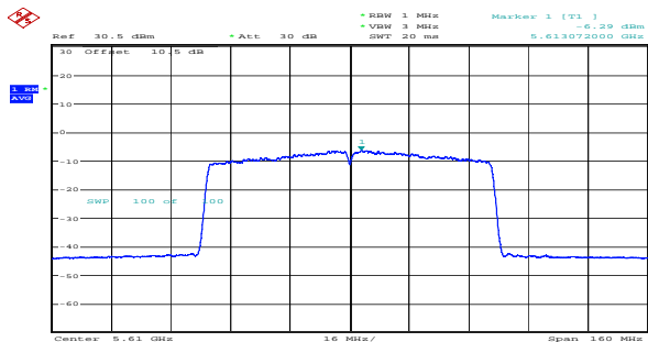
ac80_5610MHz_Chain 0 -6.29dBm/MHz
