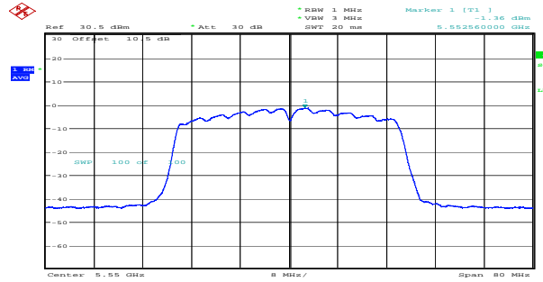
n40_5550MHz_Chain 1 -1.36dBm/MHz
