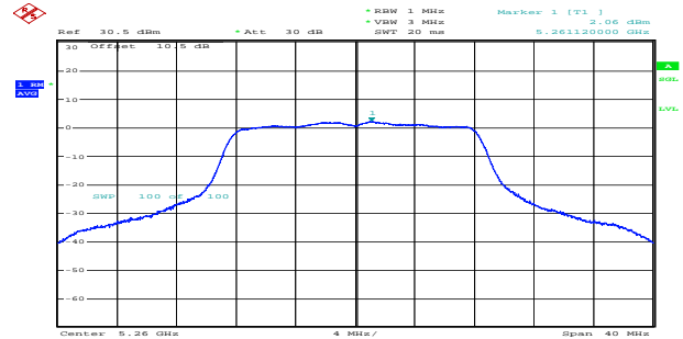
a_5260MHz_Chain 1 2.06dBm/MHz
