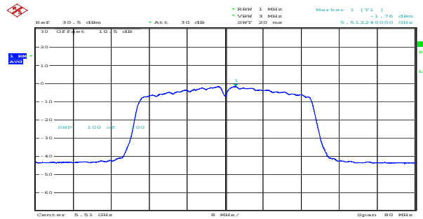
n40_5510MHz_Chain 1 -1.76dBm/MHz
