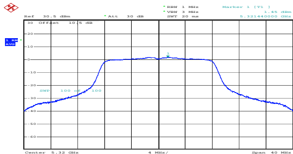
a_5320MHz_Chain 0 1.45dBm/MHz
