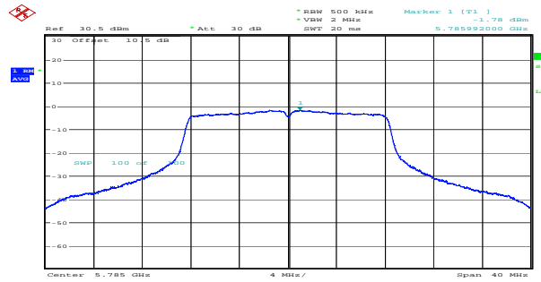
a_5785MHz_Chain 1 -1.78dBm/MHz
