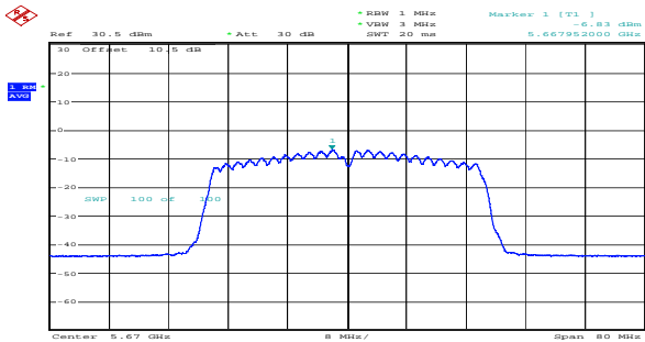
n40_5670MHz_Chain 0 -6.83dBm/MHz
