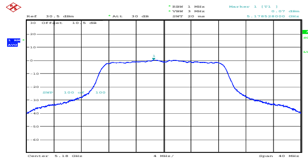
n20_5180MHz_Chain 1 0.07dBm/MHz
