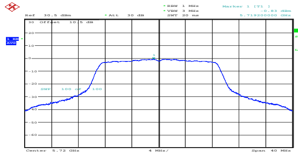
n20_5720MHz_Chain 1 -0.83dBm/MHz
