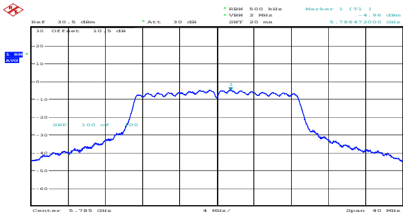
n20_5785MHz_Chain 0 -4.96dBm/MHz
