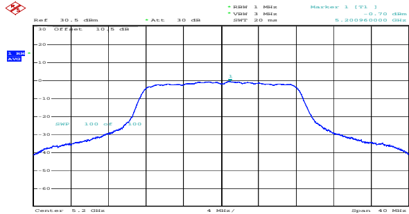
a_5200MHz_Chain 0 -0.70dBm/MHz
