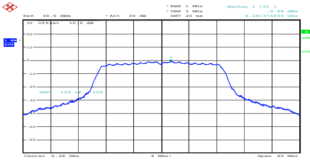
n20_5280MHz_Chain 0 -0.96dBm/MHz
