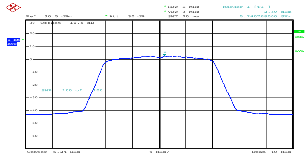
a_5240MHz_Chain 1 2.39dBm/MHz
