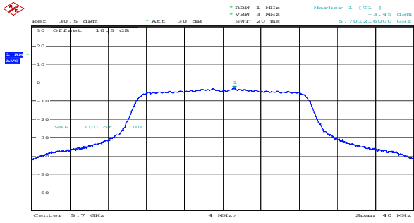
n20_5700MHz_Chain 0 -3.45dBm/MHz
