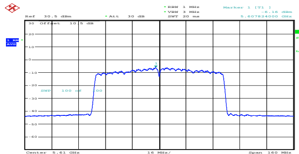
ac80_5610MHz_Chain 1 -6.16dBm/MHz
