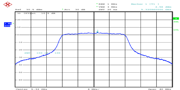
a_5320MHz_Chain 1 2.56dBm/MHz
