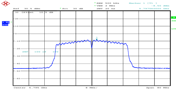
n40_5795MHz_Chain 0 -8.50dBm/MHz
