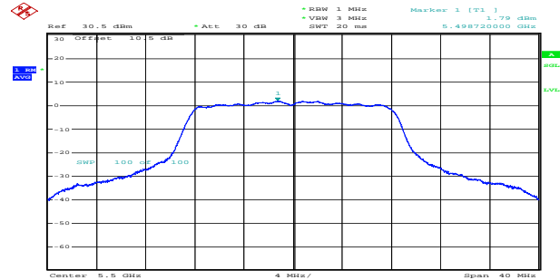
a_5500MHz_Chain 1 1.79dBm/MHz
