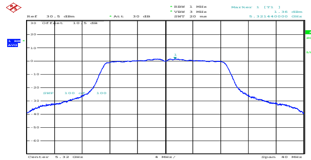
n20_5320MHz_Chain 1 1.36dBm/MHz
