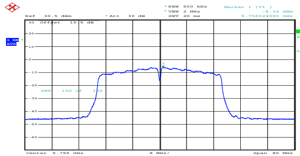
n40_5755MHz_Chain 1 -6.32dBm/MHz
