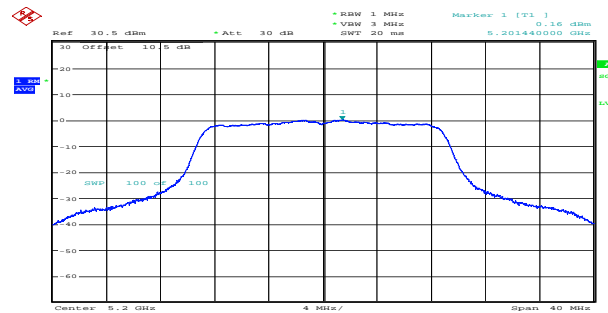
n20_5200MHz_Chain 1 0.16dBm/MHz
