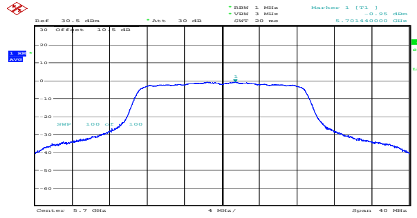
n20_5700MHz_Chain 1 -0.95dBm/MHz
