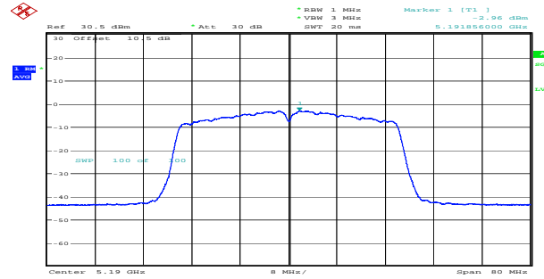
n40_5190MHz_Chain 1 -2.96dBm/MHz
