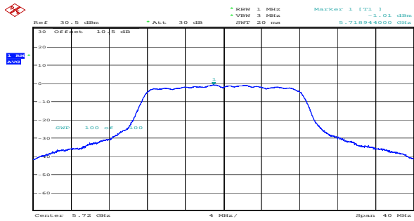
a_5720MHz_Chain 0 -1.01dBm/MHz
