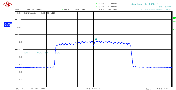
ac80_5210MHz_Chain 1 -7.98dBm/MHz
