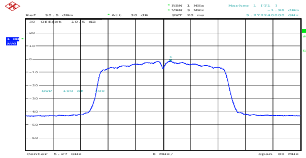
n40_5270MHz_Chain 1 -1.96dBm/MHz
