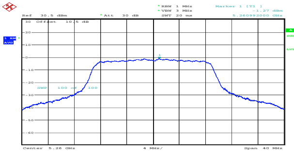
n20_5260MHz_Chain 0 -1.27dBm/MHz
