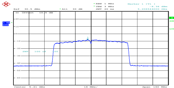
ac80_5210MHz_Chain 0 -8.36dBm/MHz
