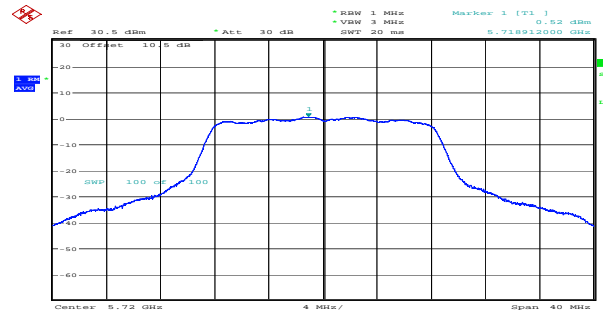
a_5720MHz_Chain 1 0.52dBm/MHz
