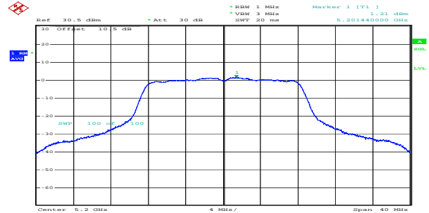
a_5200MHz_Chain 1 1.21dBm/MHz
