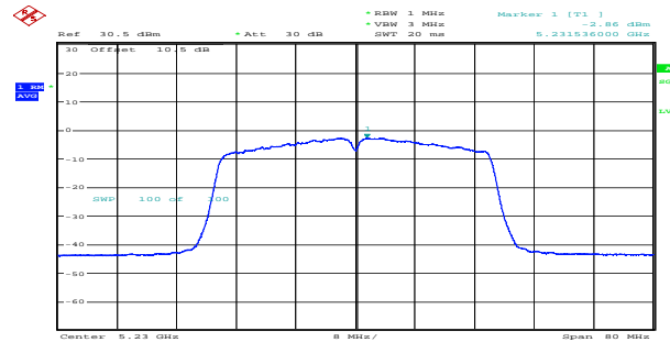
n40_5230MHz_Chain 1 -2.86dBm/MHz
