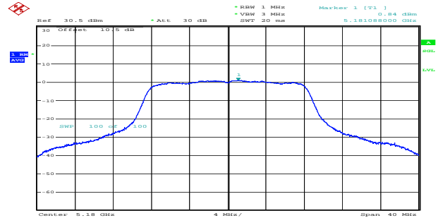
a_5180MHz_Chain 1 0.84dBm/MHz
