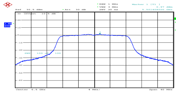
n20_5500MHz_Chain 1 0.97dBm/MHz
