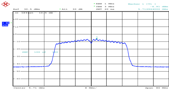
n40_5710MHz_Chain 0 -6.91dBm/MHz
