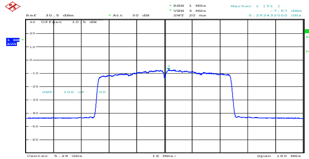
ac80_5290MHz_Chain 1 -7.57dBm/MHz
