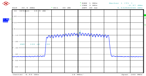
ac80_5530MHz_Chain 1 -6.57dBm/MHz
