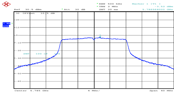
a_5785MHz_Chain 0 -3.52dBm/MHz
