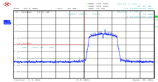
n20_2412MHz_Chain 1 42.45dB
