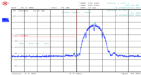
b_2412MHz_Chain 0 45.78dB
