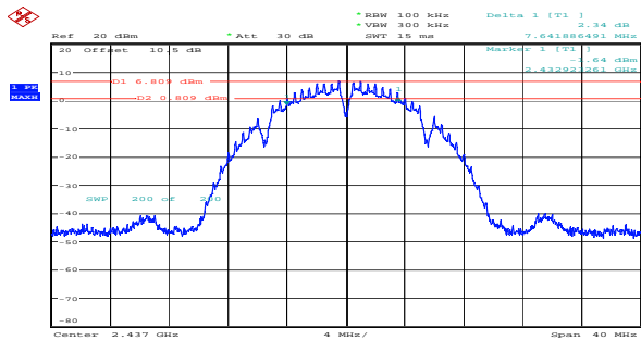
b_2437MHz_Chain 0 7.642MHz
