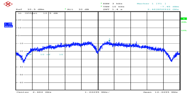
b_2462MHz_Chain 1 -7.45dBm/3kHz
