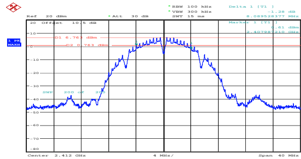
b_2412MHz_Chain 1 8.090MHz
