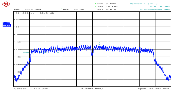
n20_2412MHz_Chain 0 -14.16dBm/3kHz
