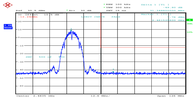
b_2462MHz_Chain 1 49.80dB
