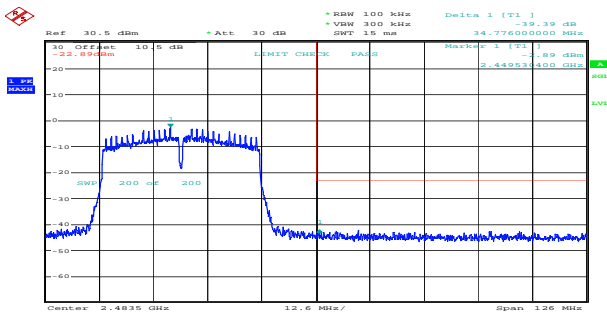
n40_2452MHz_Chain 0 39.39dB
