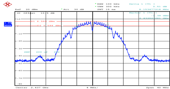
b_2437MHz_Chain 1 8.153MHz
