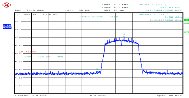
n20_2412MHz_Chain 0 42.63dB
