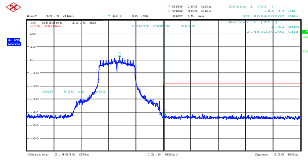
g_2462MHz_Chain 1 43.17dB
