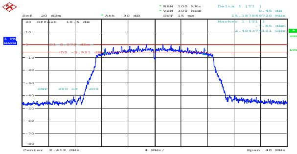
n20_2412MHz_Chain 0 15.188MHz
