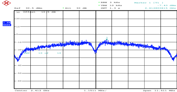
b_2412MHz_Chain 0 -7.43dBm/3kHz
