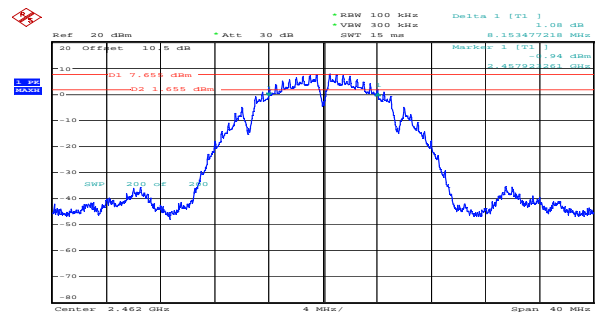
b_2462MHz_Chain 1 8.153MHz
