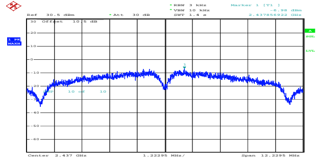
b_2437MHz_Chain 1 -6.98dBm/3kHz
