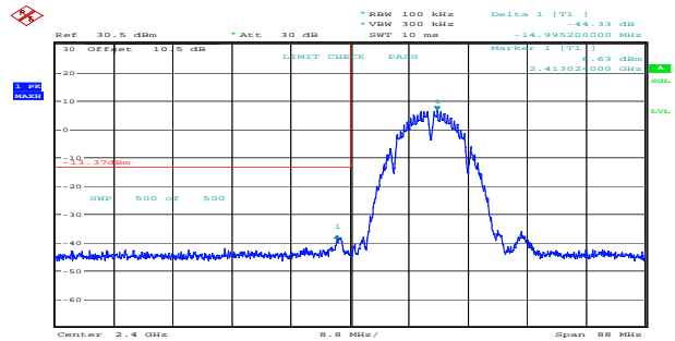
b_2412MHz_Chain 1 44.33dB
