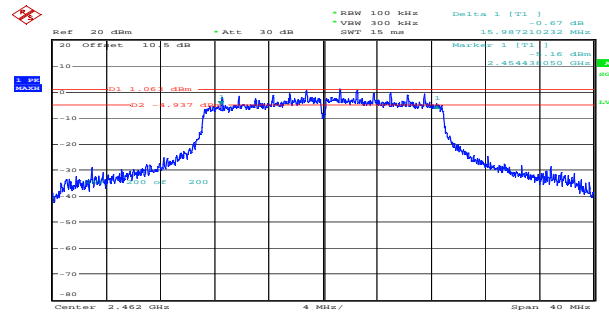
n20_2462MHz_Chain 1 15.987MHz
