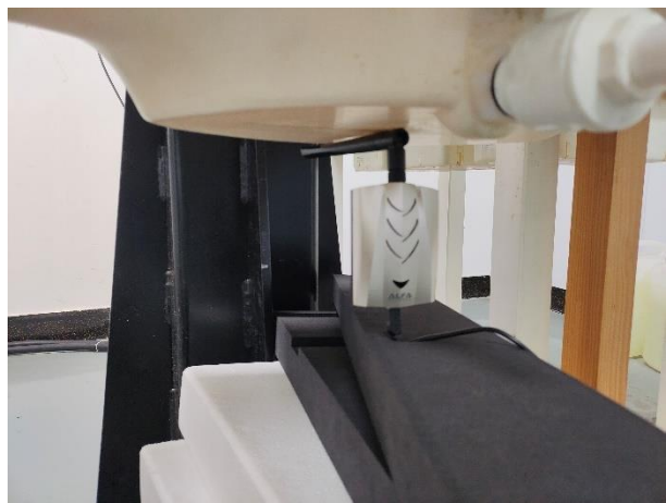
Top_Antenna Fold 90°#4
