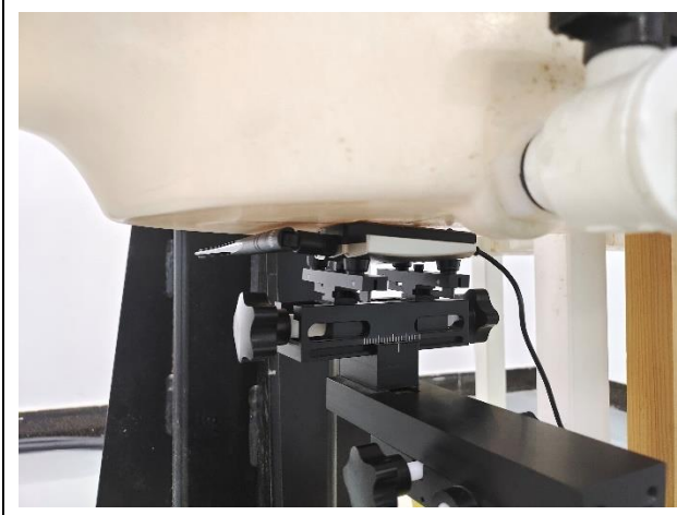
Back_Antenna Fold 90°#2
