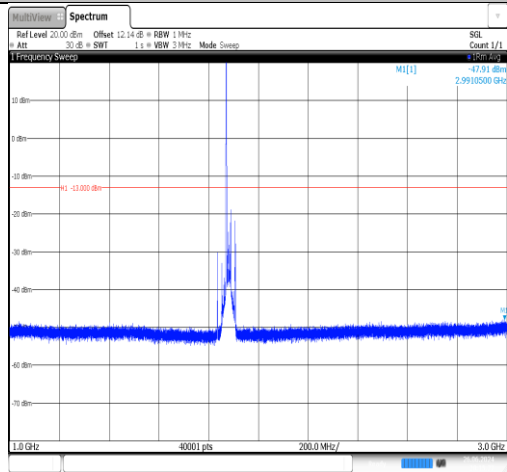
Band2-20MHz-QPSK-18900-1RB#0-1000~3000-PASS
