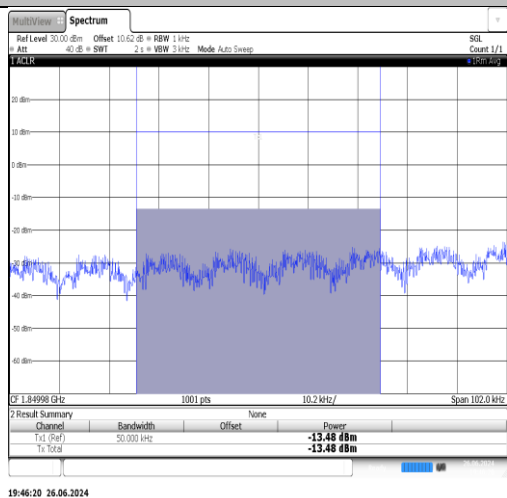
Band2-5MHz-QPSK-18625-1RB#24-PASS
