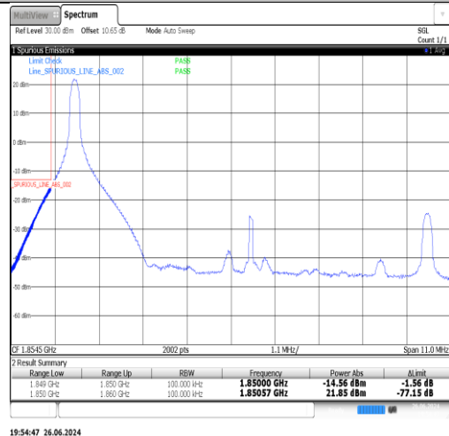
Band2-10MHz-QPSK-18650-1RB#49-PASS
