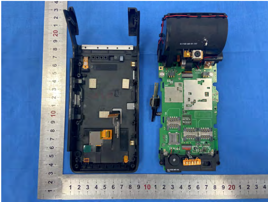
NFC antenna
