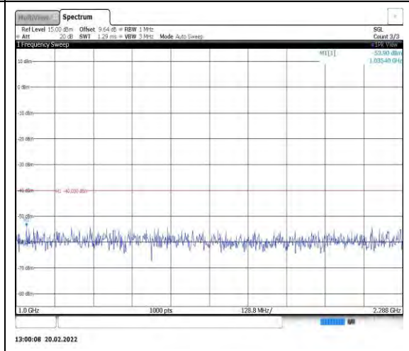
Band40-5MHz-16QAM-39200-1RB#0- Range2:1000~2288MHz
