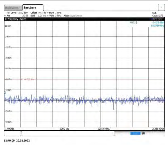
Band40-5MHz-16QAM-38725-1RB#0- Range2:1000~2288MHz
