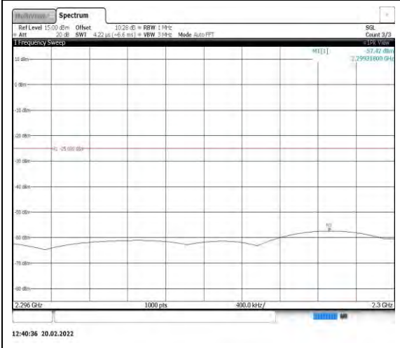
Band40-5MHz-16QAM-38725-1RB#0- Range5:2296~2300MHz
