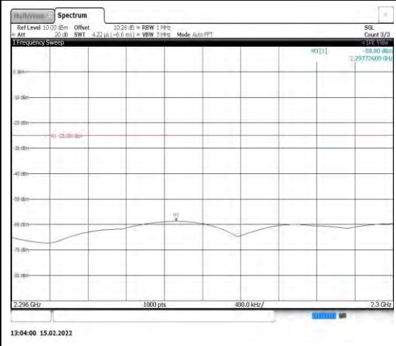
Band40-10MHz-QPSK-39200-1RB#0- Range5:2296~2300MHz
