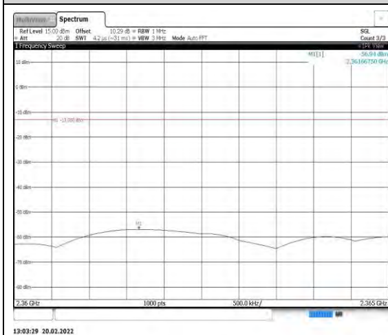
Band40-5MHz-QPSK-39225-1RB#0- Range12:2360~2365MHz
