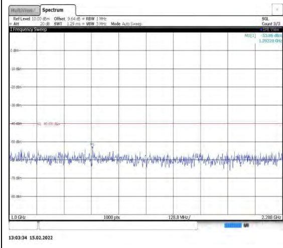
Band40-10MHz-QPSK-39200-1RB#0- Range2:1000~2288MHz
