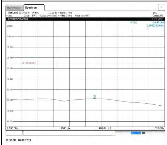
Band40-10MHz-QPSK-38750-1RB#0- Range5:2296~2300MHz
