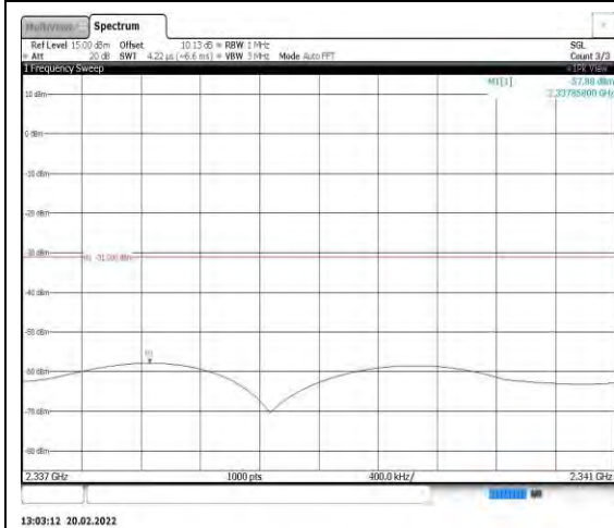
Band40-5MHz-QPSK-39225-1RB#0- Range10:2337~2341MHz
