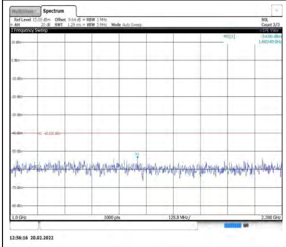
Band40-5MHz-16QAM-39175-1RB#0- Range2:1000~2288MHz
