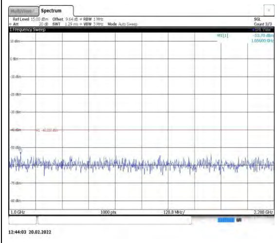
Band40-5MHz-16QAM-38750-1RB#0- Range2:1000~2288MHz
