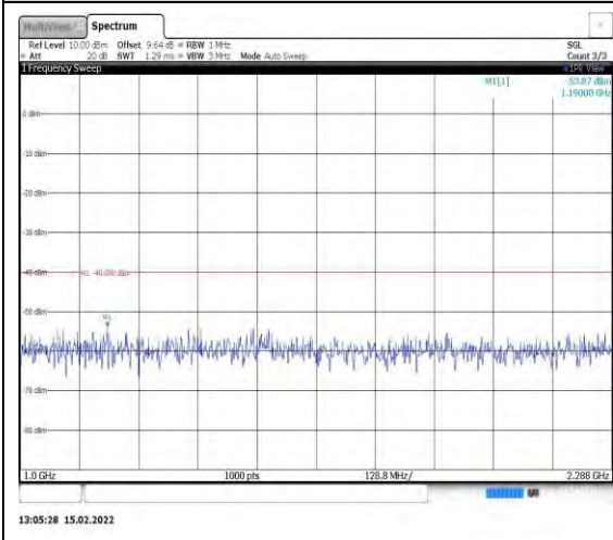
Band40-10MHz-16QAM-39200-1RB#0- Range2:1000~2288MHz
