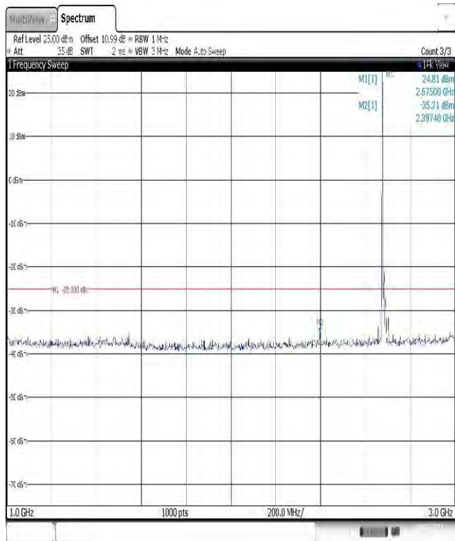
Band41-15MHz-QPSK-41515-1RB#0-Range2:1000~3000MHz
