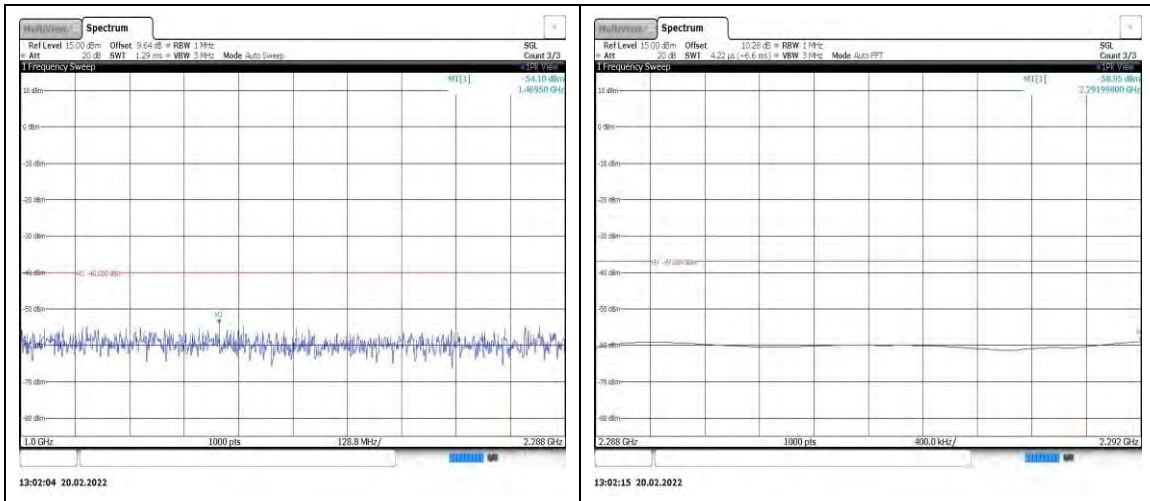
Band40-5MHz-QPSK-39225-1RB#0- Range2:1000~2288MHz
