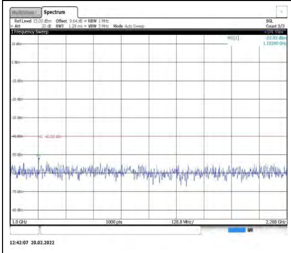
Band40-5MHz-QPSK-38750-1RB#0- Range2:1000~2288MHz
