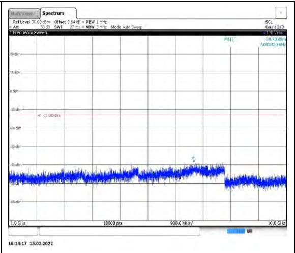
Band26-1.4MHz-QPSK-26697-1RB#0- Range2:1000~10000MHz
