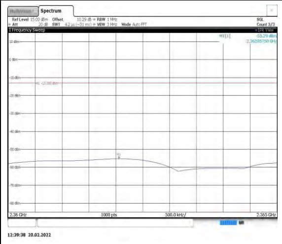
Band40-5MHz-QPSK-38725-1RB#0- Range12:2360~2365MHz
