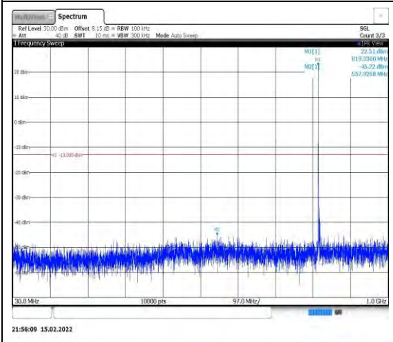
Band26-5MHz-QPSK-26765-1RB#0- Range1:30~1000MHz
