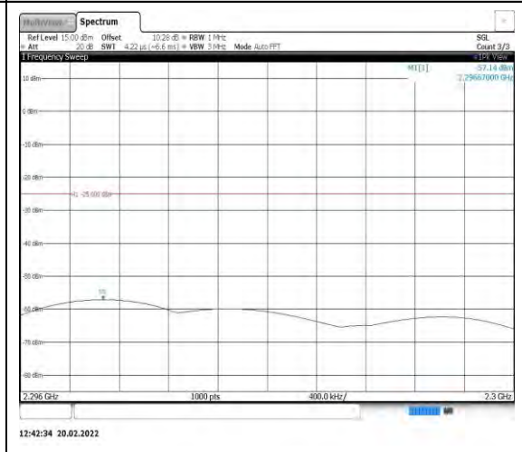
Band40-5MHz-QPSK-38750-1RB#0- Range5:2296~2300MHz
