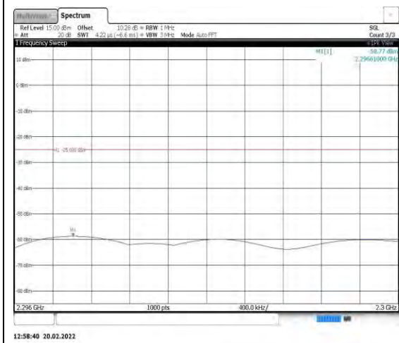
Band40-5MHz-QPSK-39200-1RB#0- Range5:2296~2300MHz
