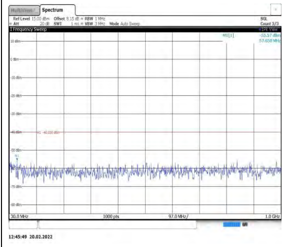
Band40-5MHz-QPSK-38775-1RB#0- Range1:30~1000MHz
