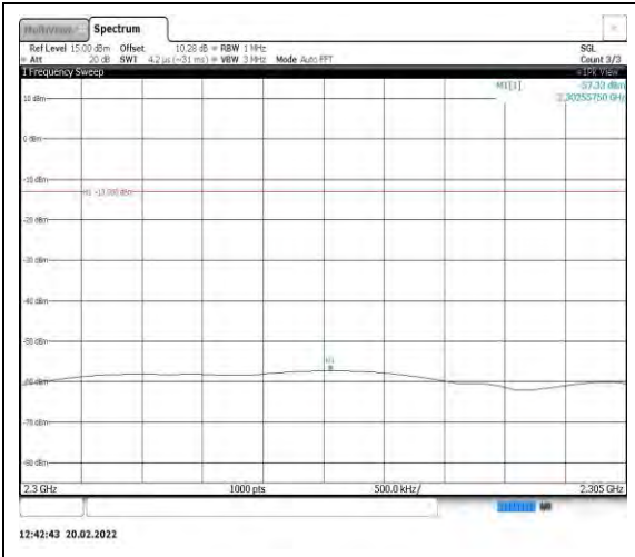
Band40-5MHz-QPSK-38750-1RB#0- Range6:2300~2305MHz
