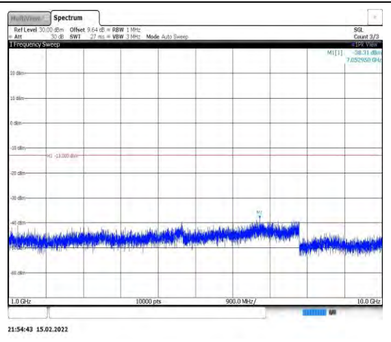
Band26-5MHz-QPSK-26715-1RB#0- Range2:1000~10000MHz
