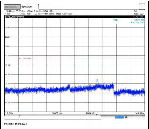
Band26-1.4MHz-QPSK-26797-1RB#0- Range2:1000~10000MHz
