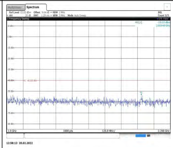
Band40-5MHz-QPSK-39200-1RB#0- Range2:1000~2288MHz
