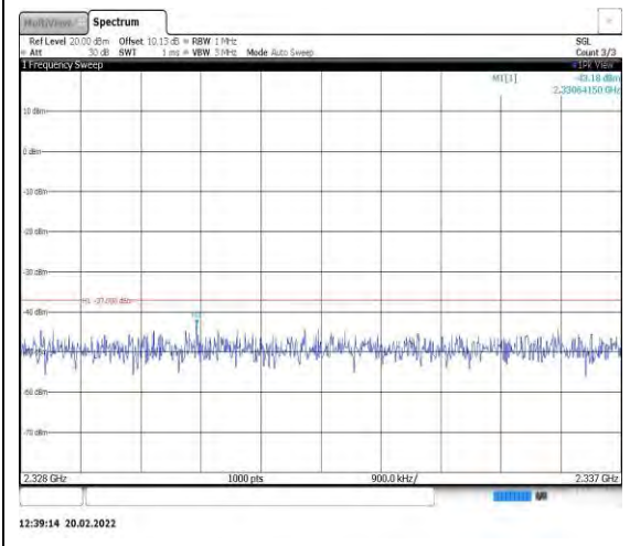
Band40-5MHz-QPSK-38725-1RB#0- Range9:2328~2337MHz
