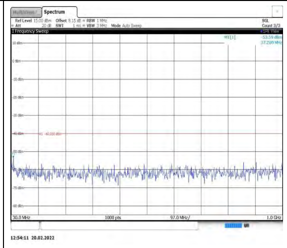
Band40-5MHz-QPSK-39175-1RB#0- Range1:30~1000MHz
