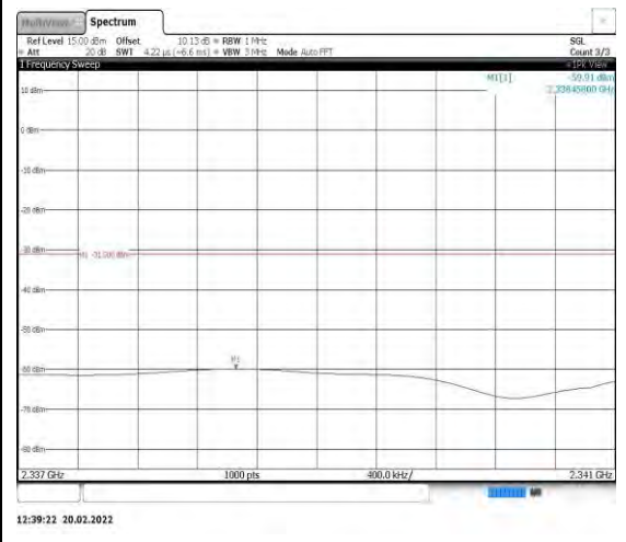
Band40-5MHz-QPSK-38725-1RB#0- Range10:2337~2341MHz
