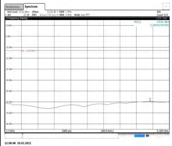
Band40-5MHz-QPSK-39200-1RB#0- Range6:2300~2305MHz
