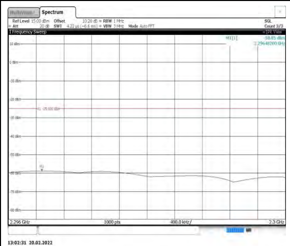
Band40-5MHz-QPSK-39225-1RB#0- Range5:2296~2300MHz
