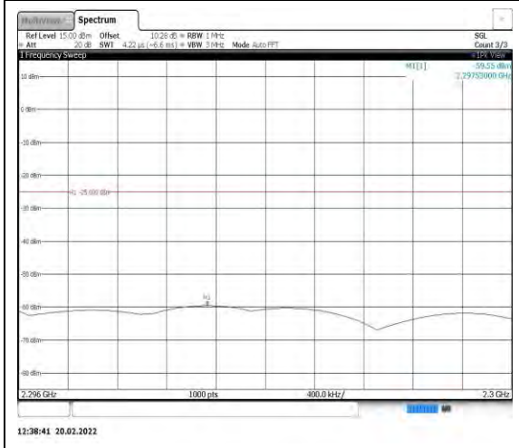
Band40-5MHz-QPSK-38725-1RB#0- Range5:2296~2300MHz
