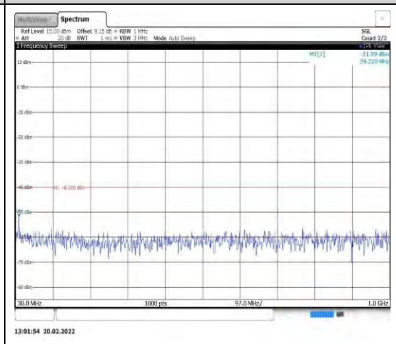
Band40-5MHz-QPSK-39225-1RB#0- Range1:30~1000MHz
