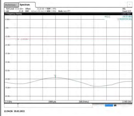
Band40-5MHz-QPSK-39175-1RB#0- Range6:2300~2305MHz
