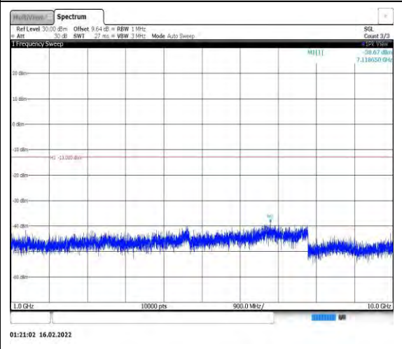
Band26-3MHz-QPSK-27025-1RB#0- Range2:1000~10000MHz
