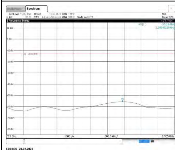
Band40-5MHz-QPSK-39225-1RB#0- Range6:2300~2305MHz
