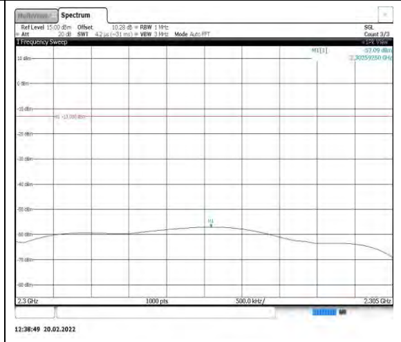
Band40-5MHz-QPSK-38725-1RB#0- Range6:2300~2305MHz
