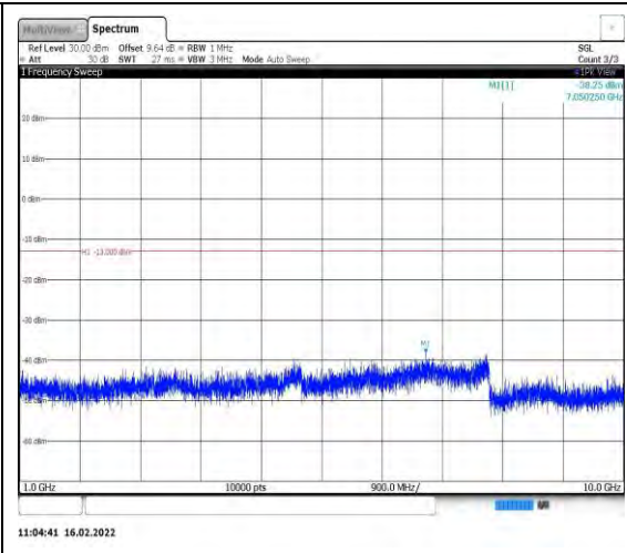
Band26-10MHz-QPSK-26990-1RB#0- Range2:1000~10000MHz
