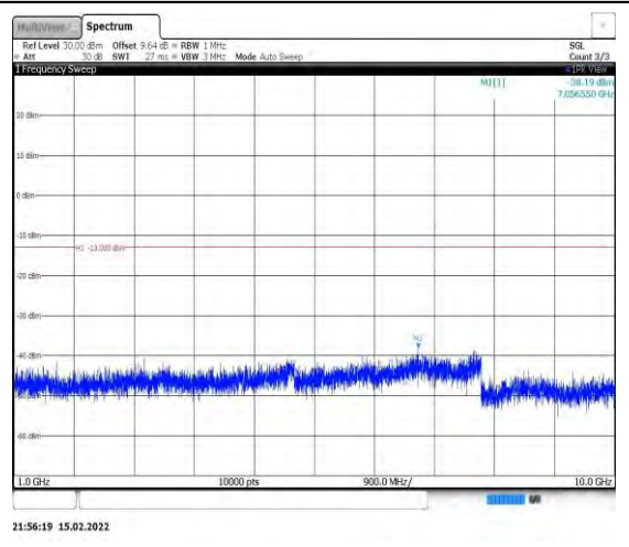
Band26-5MHz-QPSK-26765-1RB#0- Range2:1000~10000MHz
