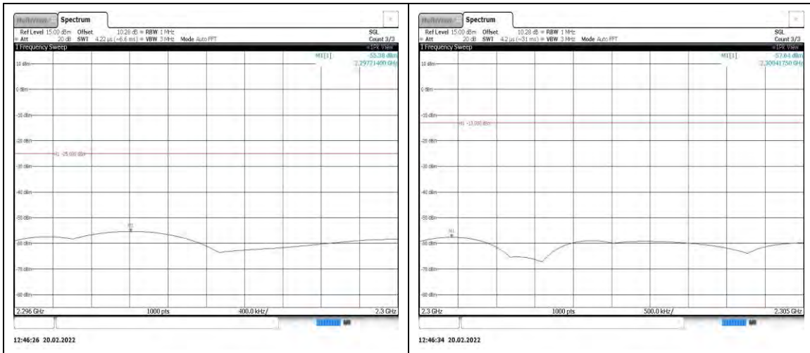
Band40-5MHz-QPSK-38775-1RB#0- Range5:2296~2300MHz
