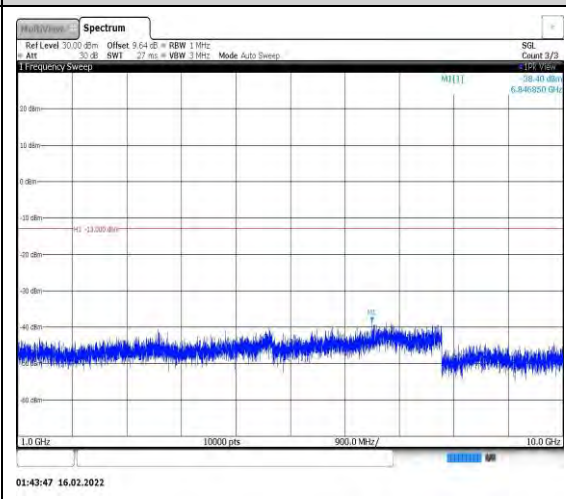
Band26-5MHz-QPSK-27015-1RB#0- Range2:1000~10000MHz
