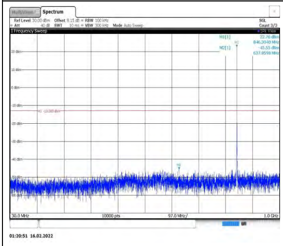
Band26-3MHz-QPSK-27025-1RB#0- Range1:30~1000MHz
