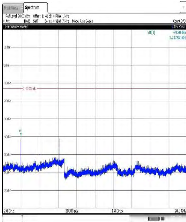
Band25-20MHz-QPSK-26365-1RB#0-Range3:2000~20000MHz
