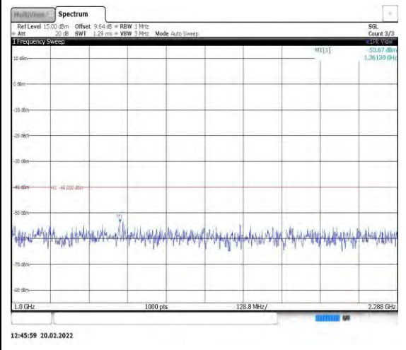
Band40-5MHz-QPSK-38775-1RB#0- Range2:1000~2288MHz
