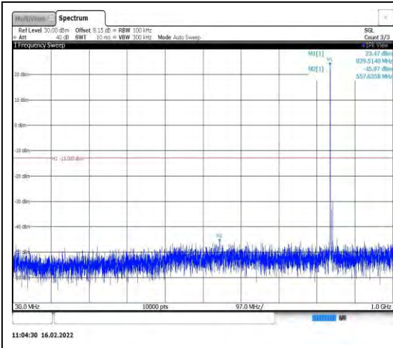
Band26-10MHz-QPSK-26990-1RB#0- Range1:30~1000MHz
