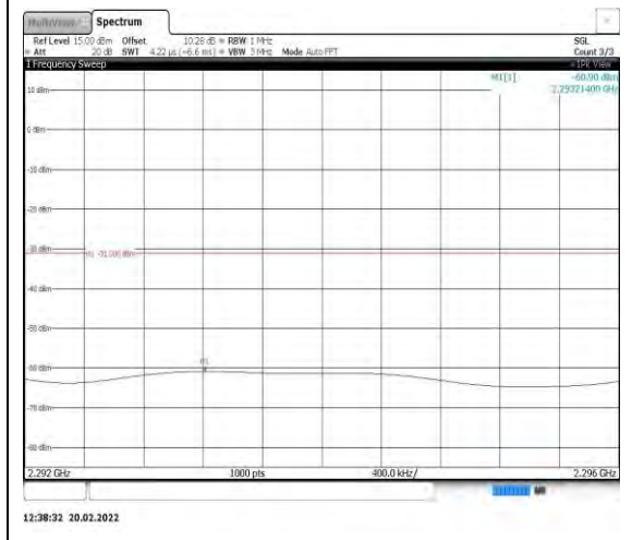
Band40-5MHz-QPSK-38725-1RB#0- Range4:2292~2296MHz
