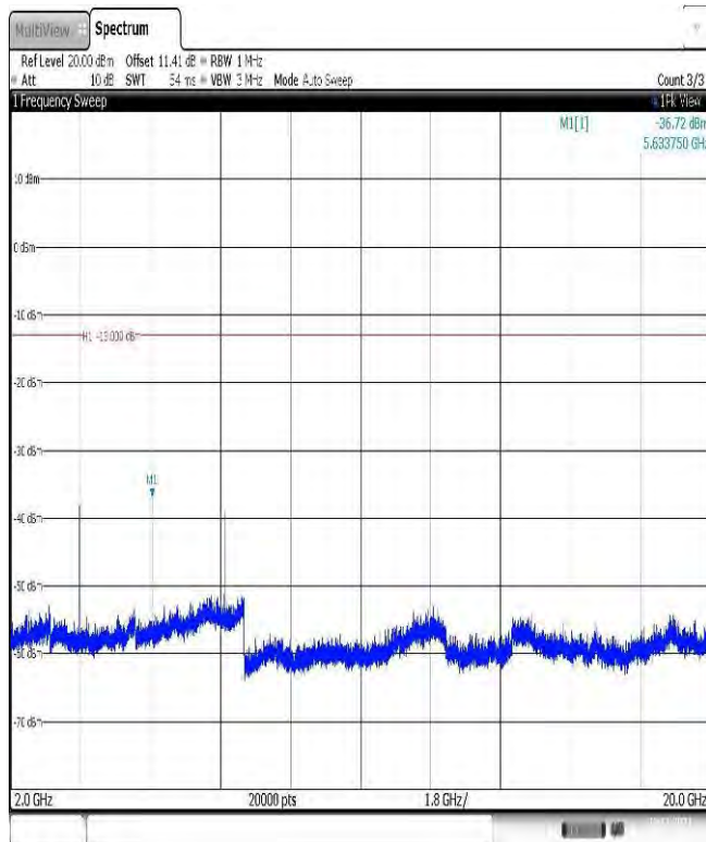
Band25-10MHz-QPSK-26365-1RB#0-Range3:2000~20000MHz
