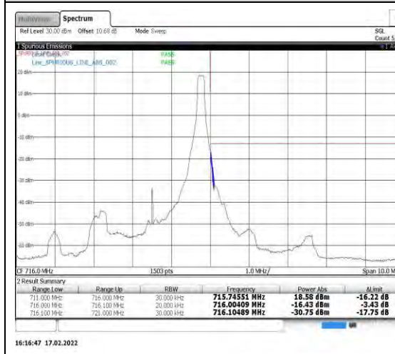
Band12-3MHz-QPSK-23165-1RB#14
