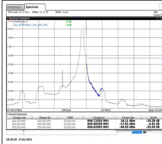
Band5-3MHz-QPSK-20635-1RB#14
