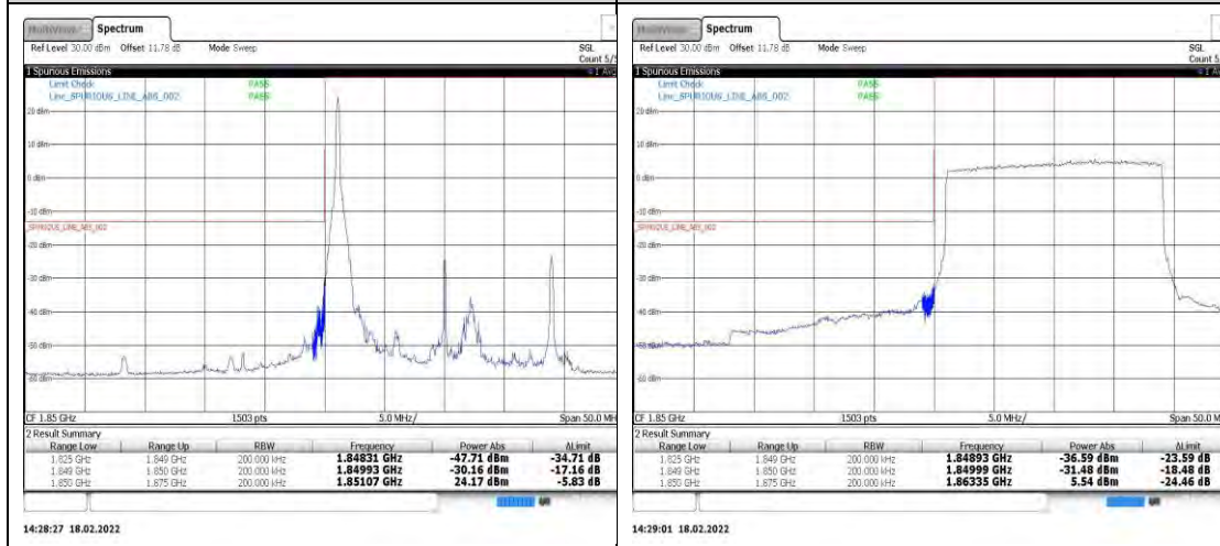
Band2-20MHz-QPSK-18700-1RB#0
