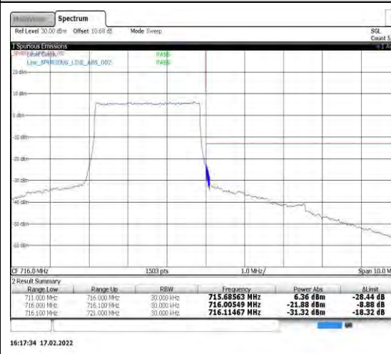
Band12-3MHz-QPSK-23165-15RB#0
