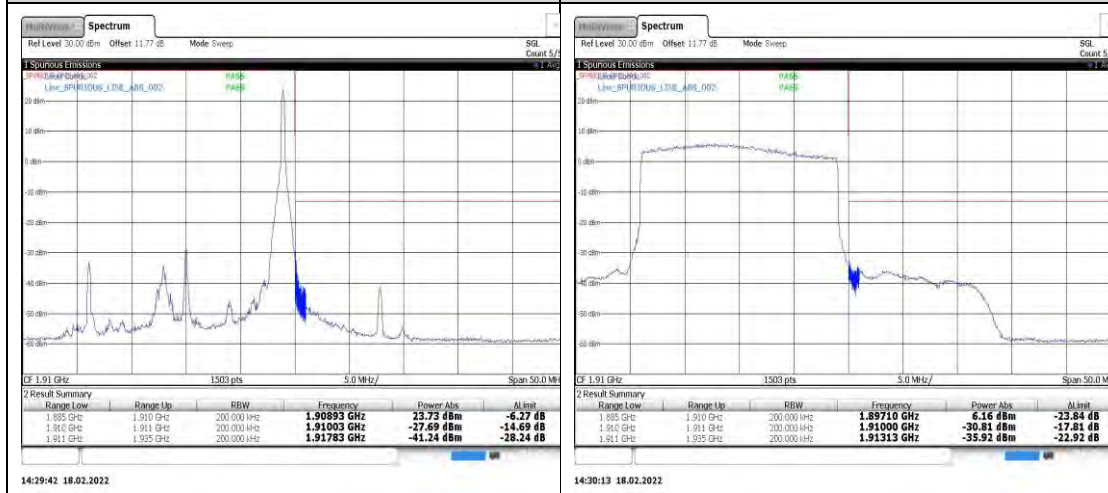
Band2-20MHz-QPSK-19100-1RB#99
