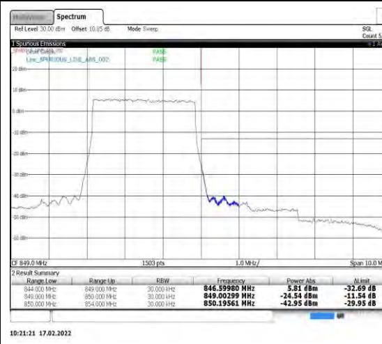
Band5-3MHz-QPSK-20635-15RB#0
