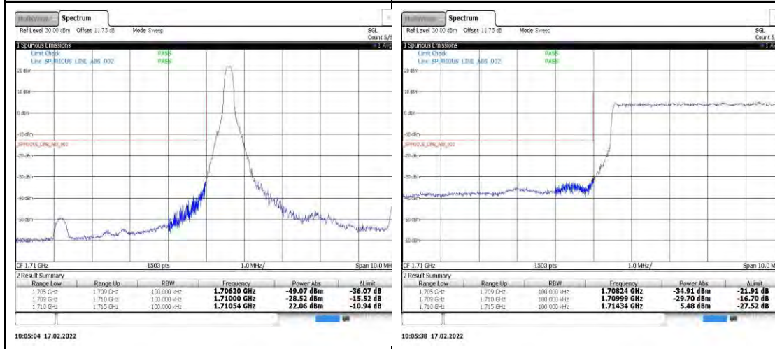
Band4-10MHz-QPSK-20000-1RB#0
