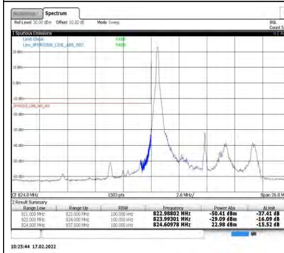
Band5-10MHz-QPSK-20450-1RB#0
