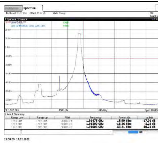
Band25-3MHz-QPSK-26675-1RB#14
