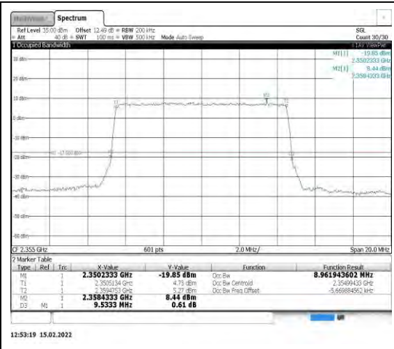
Band40-10MHz-QPSK-39200-50RB#0
