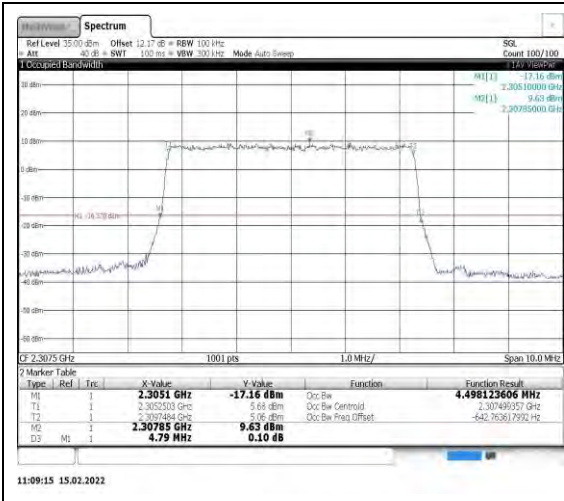
Band40-5MHz-QPSK-38725-25RB#0
