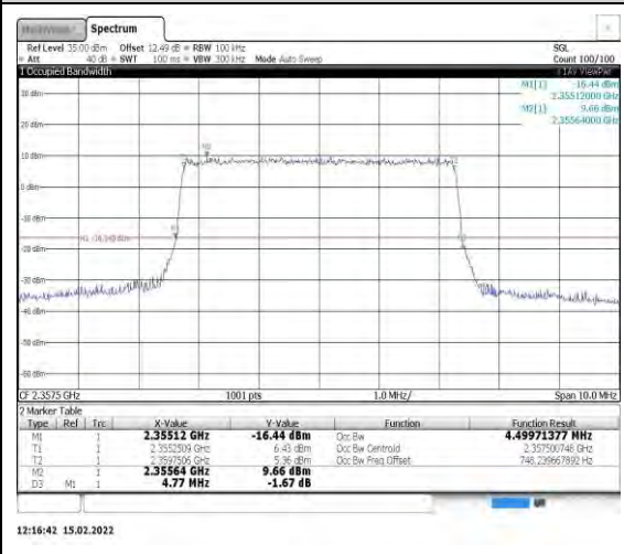
Band40-5MHz-QPSK-39225-25RB#0
