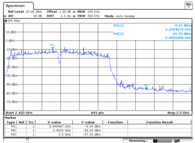
CH09-Bandedge
