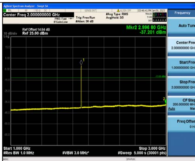
Band2-9538-2-3000~10000MHz
