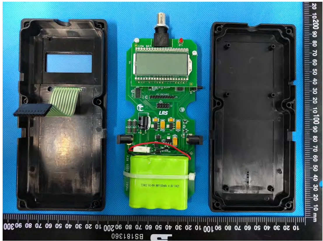
Model: TX-9561EZ
