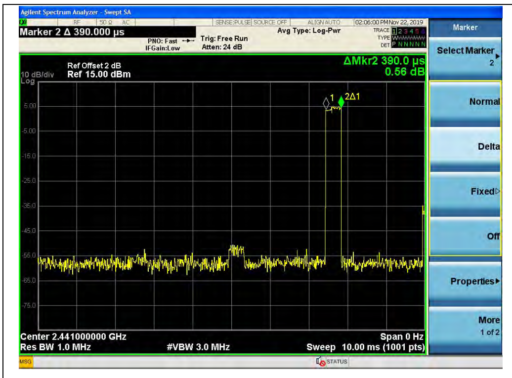
(DH1, 8-DPSK)
