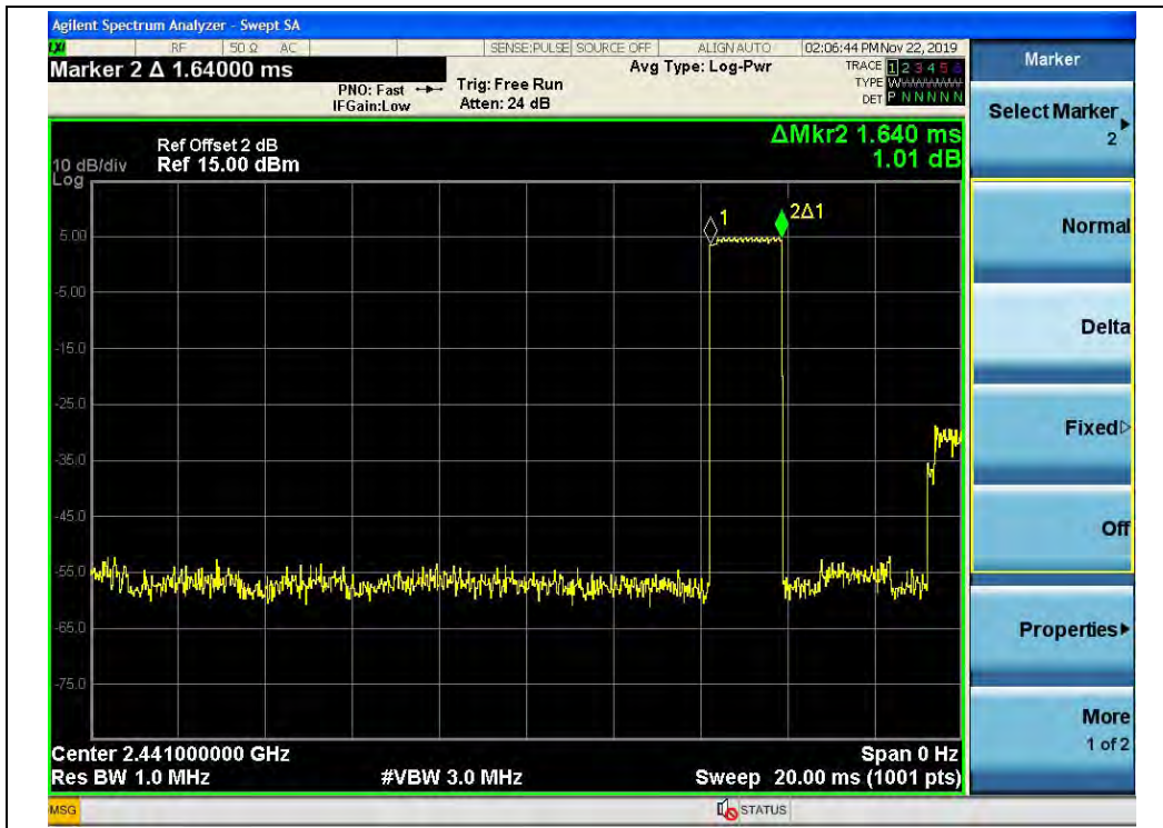
(DH3, 8-DPSK)
