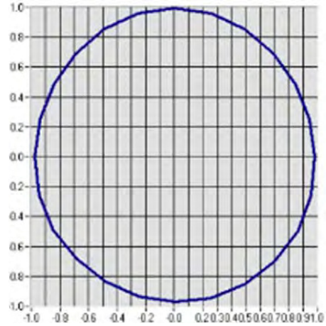
Isotropy @ 1900MHz
