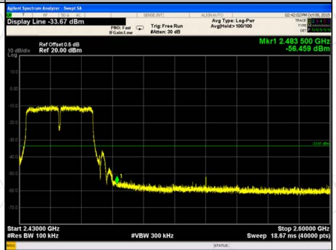
Band Edge
