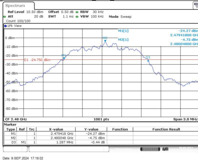
2DH5_Ant1_2480
