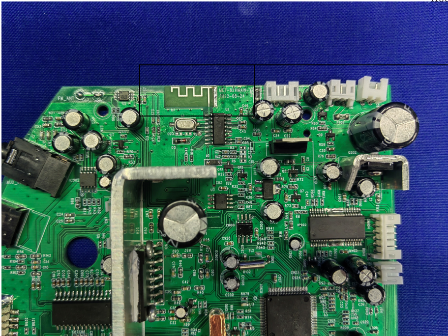
PCB ant
