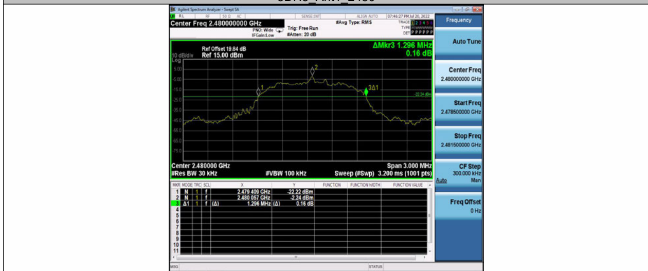
3DH5 Ant1 2480
