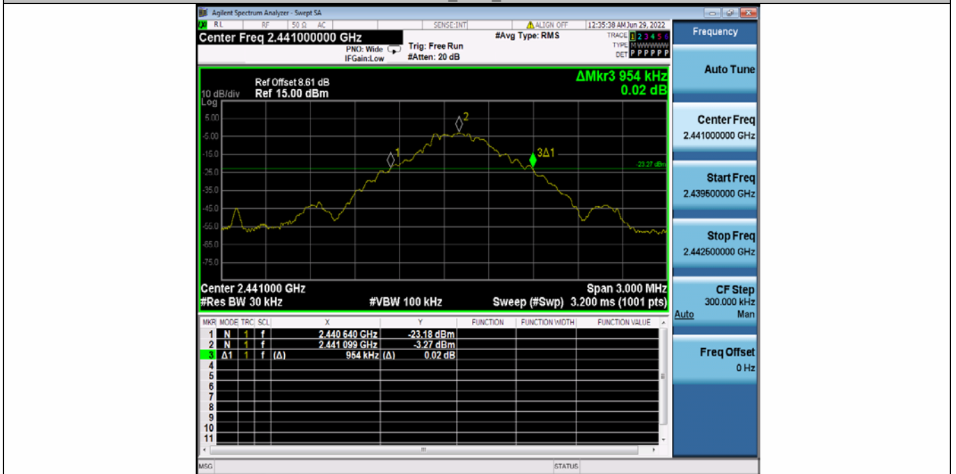
DH5_Ant1_2441
