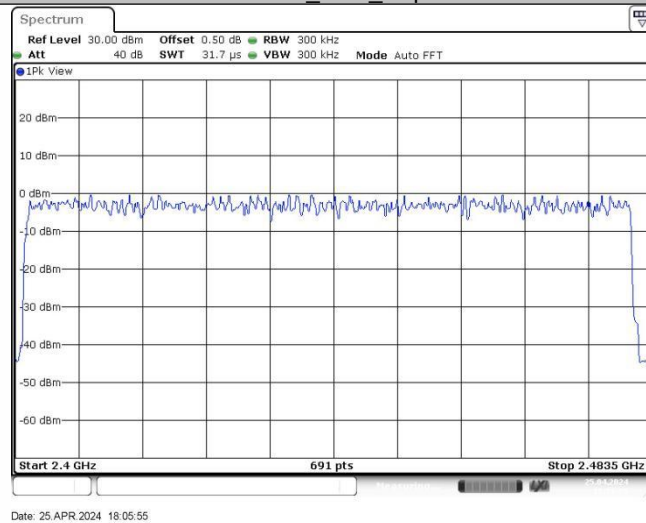
3DH5_Ant1_Hop
