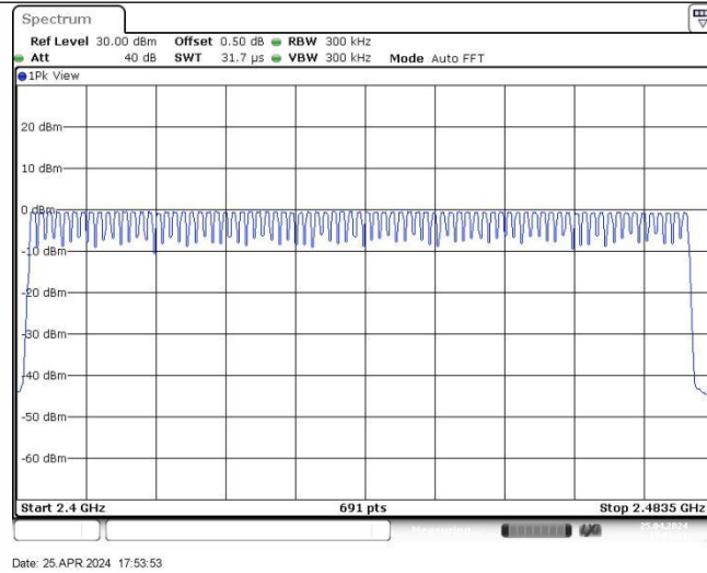
DH5_Ant1_Hop
