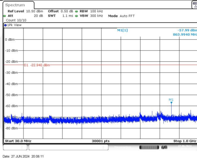
DH5_Ant1_2480_30-1000
