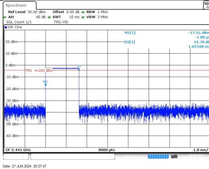
DH3_Ant1_Hop
