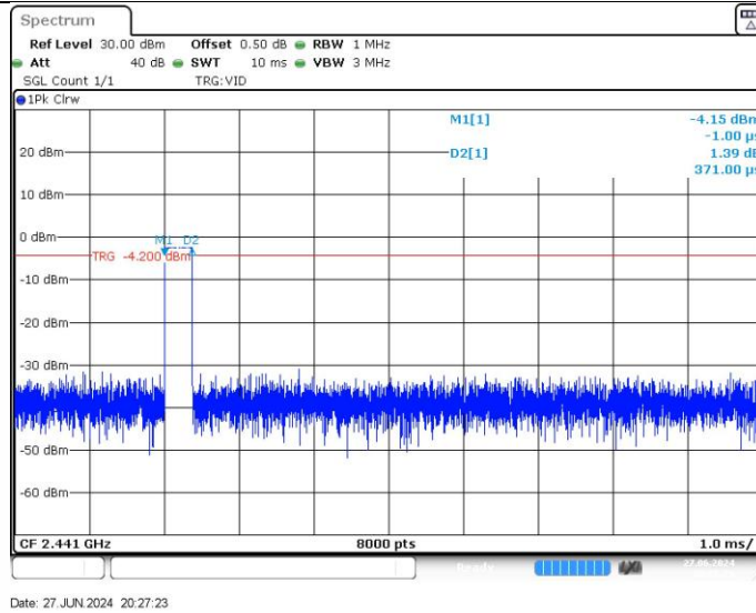
DH1_Ant1_Hop
