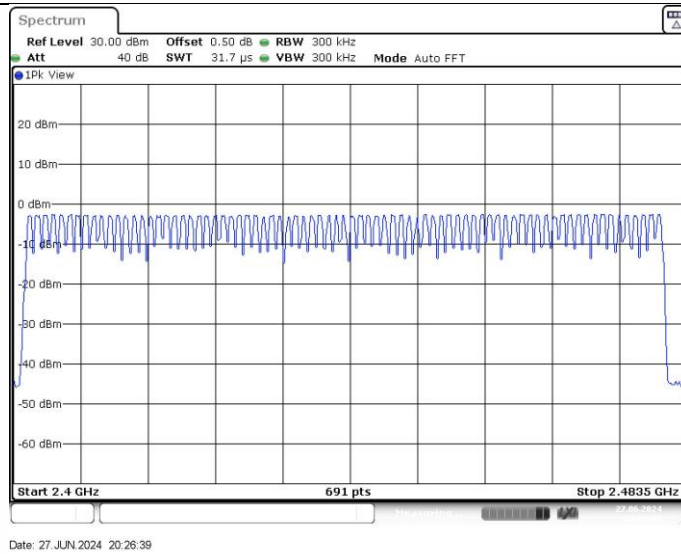
DH5_Ant1_Hop
