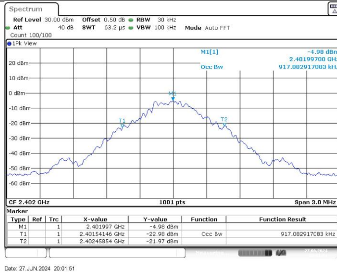
DH5_Ant1_2402
