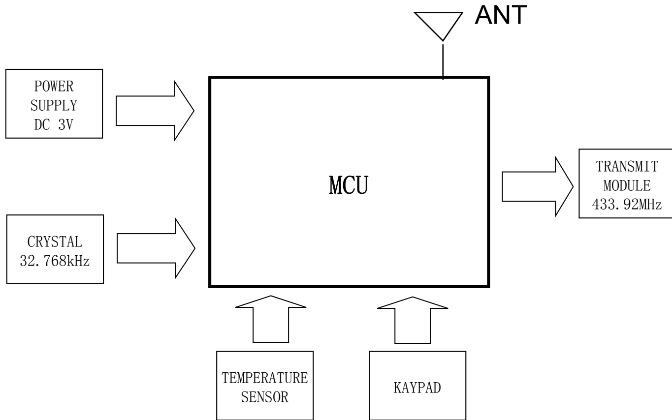
IC6008,7600(TX) BLOCK DIAGRAM
