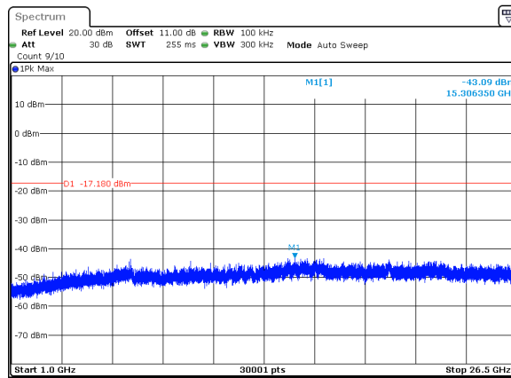
Zigbee_Ant1_2405_1000~26500
