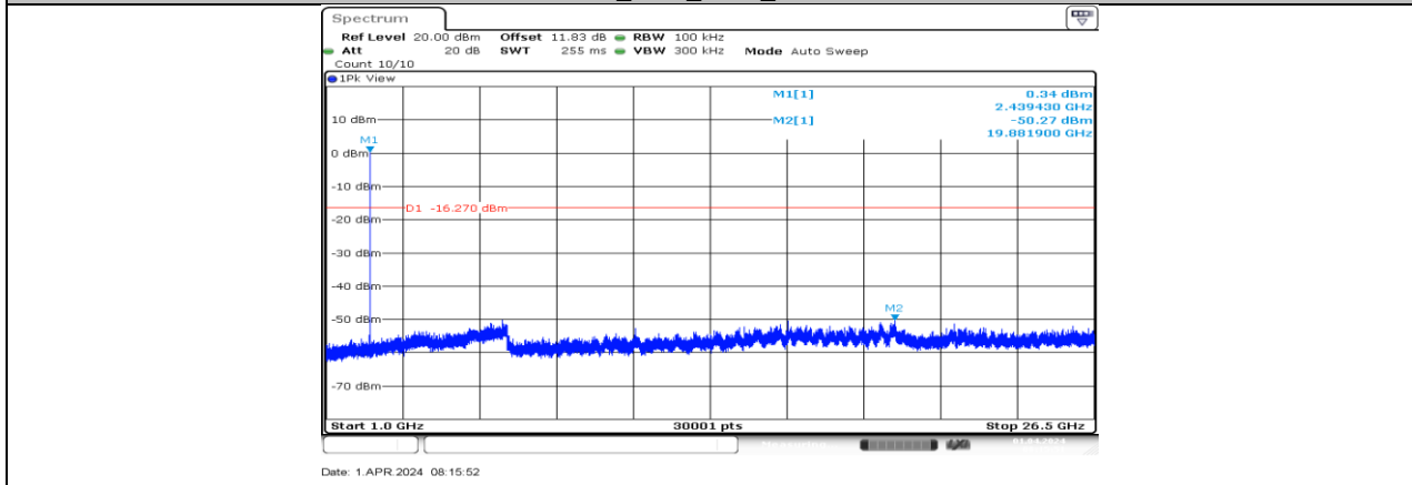
LE 2M_Ant1_2440_1000~26500
