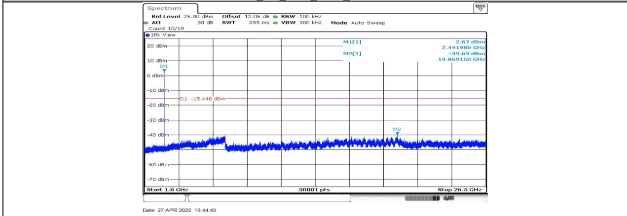
BLE_2M_Ant1_2442_1000~26500
