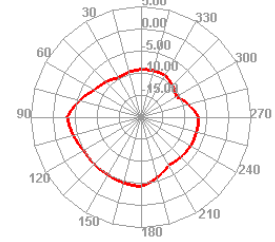
2450.000MHz E2
