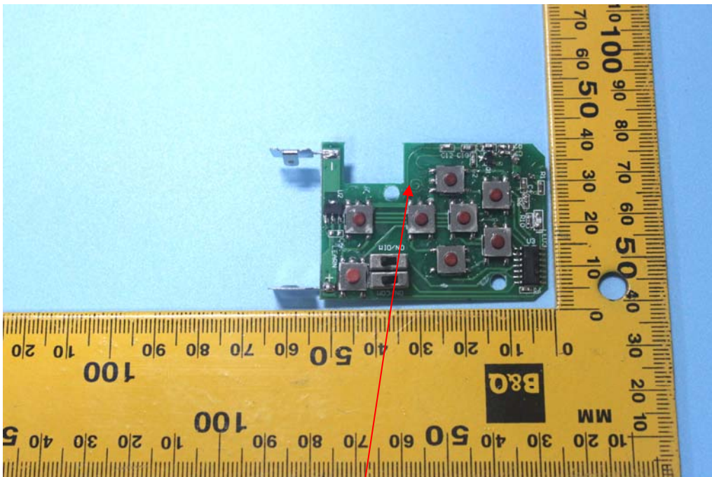
Antenna
